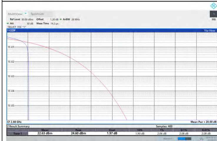
Band41-20MHz-64QAM-41490-1RB#0
