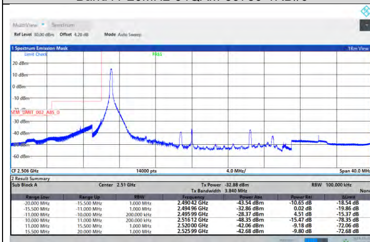
Band41-20MHz-64QAM-41490-1RB#99
