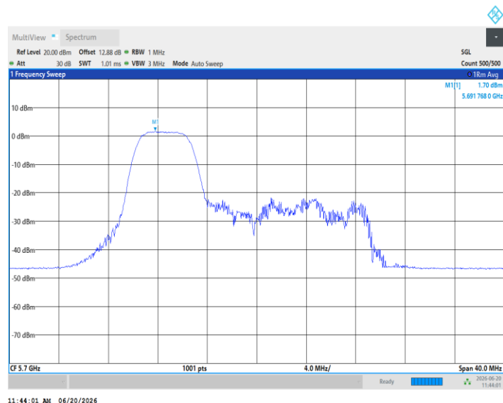
11AX20MIMO_Ant5_5700_52Tone_RU38
