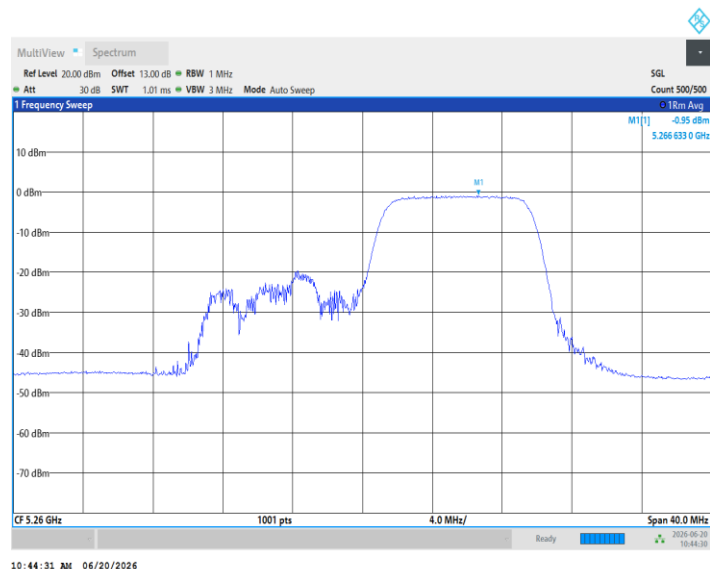
11AX20MIMO_Ant5_5260_26Tone_RU0
