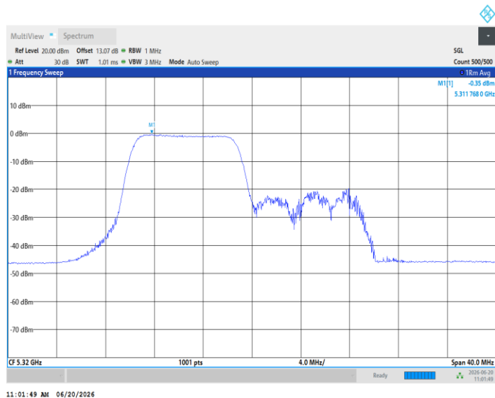
11AX20MIMO_Ant5_5320_106Tone_RU54
