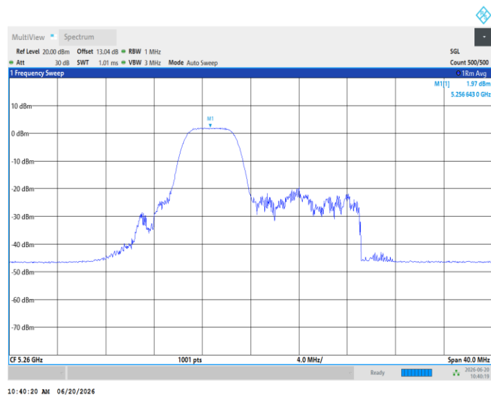
11AX20MIMO_Ant5_5260_52Tone_RU40
