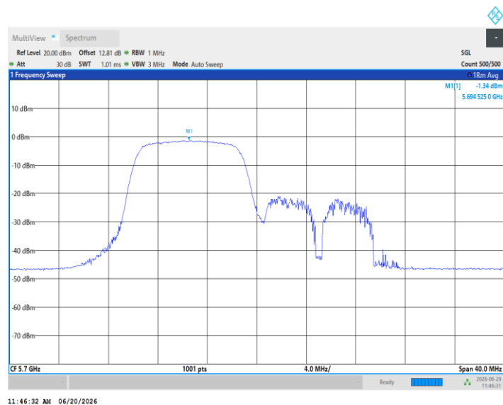
11AX20MIMO_Ant3_5700_106Tone_RU54
