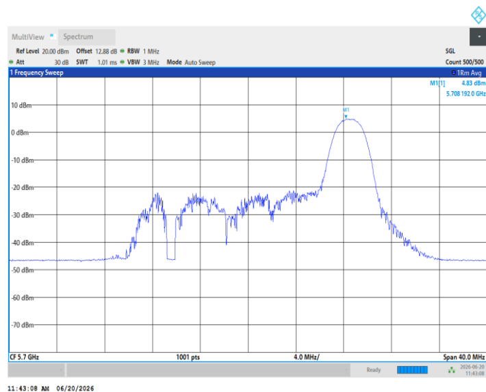
11AX20MIMO_Ant5_5700_52Tone_RU37
