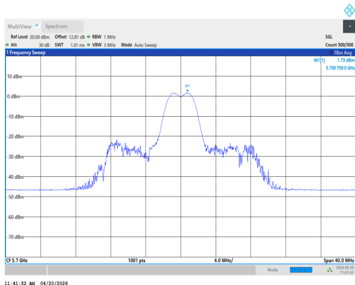
11AX20MIMO_Ant3_5700_26Tone_RU8
