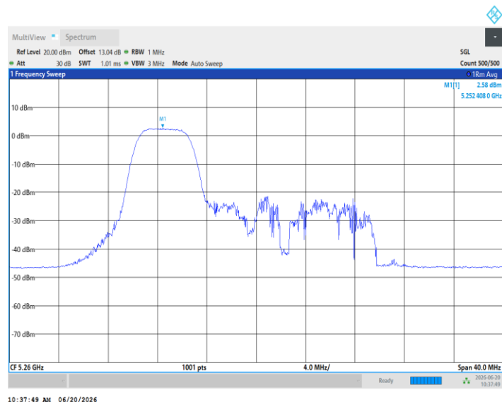
11AX20MIMO_Ant5_5260_52Tone_RU38
