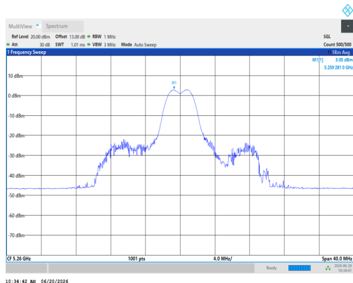
11AX20MIMO_Ant3_5260_26Tone_RU8
