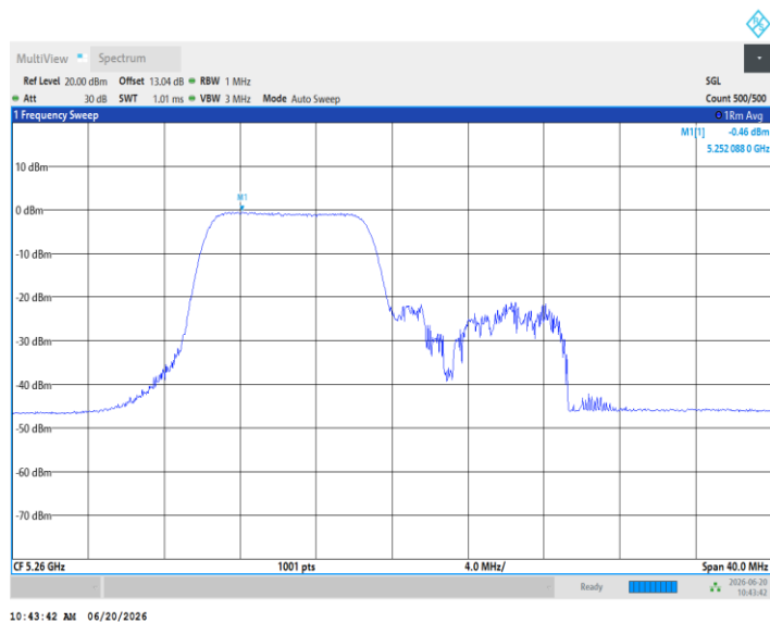
11AX20MIMO_Ant5_5260_106Tone_RU54
