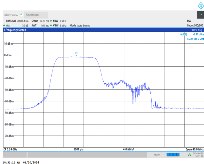
11AX20MIMO_Ant3_5240_106Tone_RU54
