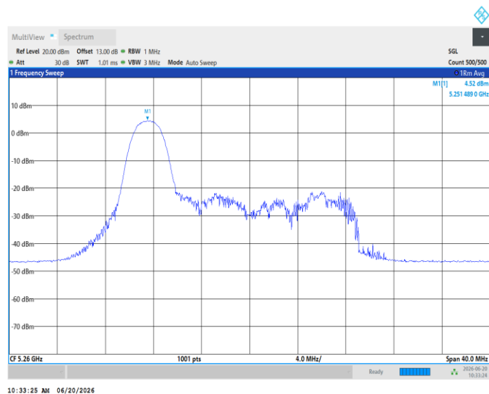
11AX20MIMO_Ant3_5260_26Tone_RU4
