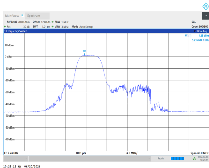
11AX20MIMO_Ant3_5240_52Tone_RU40
