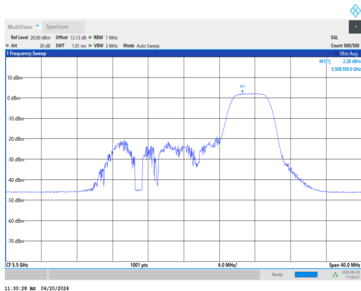
11AX20MIMO_Ant5_5500_106Tone_RU53
