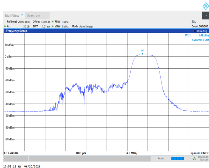
11AX20MIMO_Ant3_5280_106Tone_RU53
