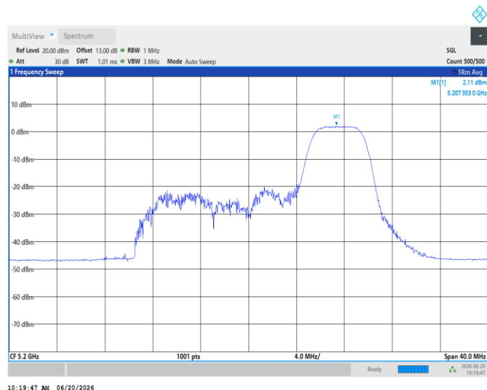
11AX20MIMO_Ant5_5200_106Tone_RU53
