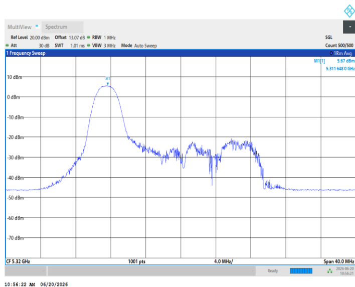
11AX20MIMO_Ant5_5320_26Tone_RU4
