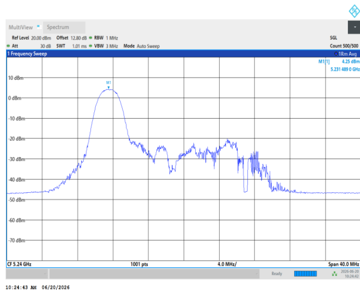
11AX20MIMO_Ant3_5240_26Tone_RU4
