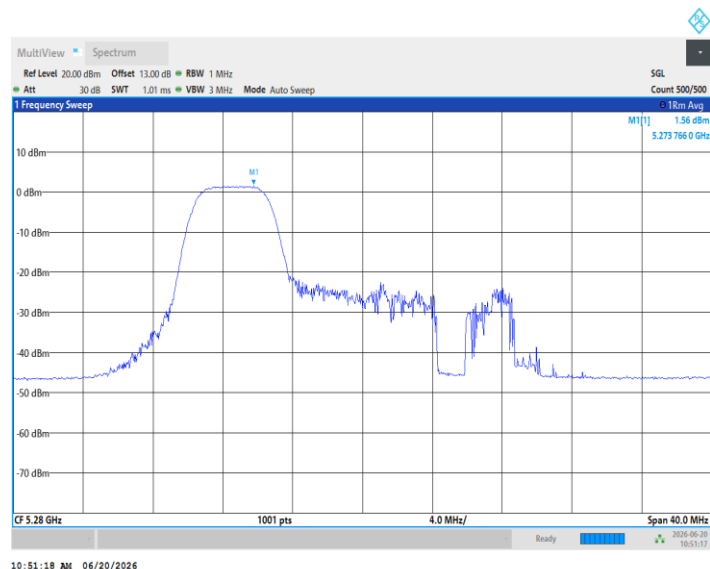
11AX20MIMO_Ant3_5280_52Tone_RU38
