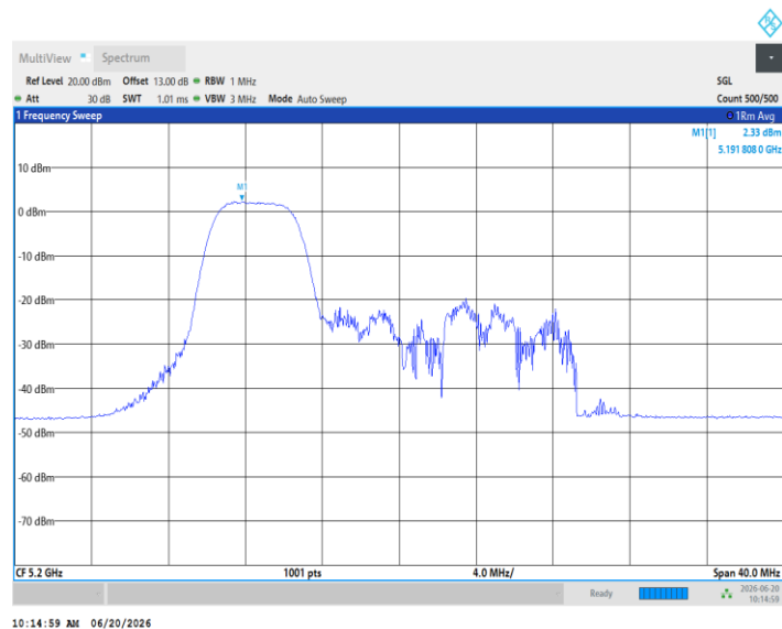
11AX20MIMO_Ant5_5200_52Tone_RU38
