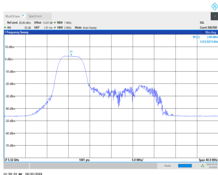
11AX20MIMO_Ant5_5320_52Tone_RU38
