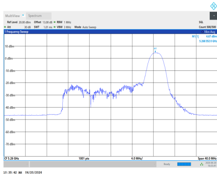
11AX20MIMO_Ant3_5260_52Tone_RU37
