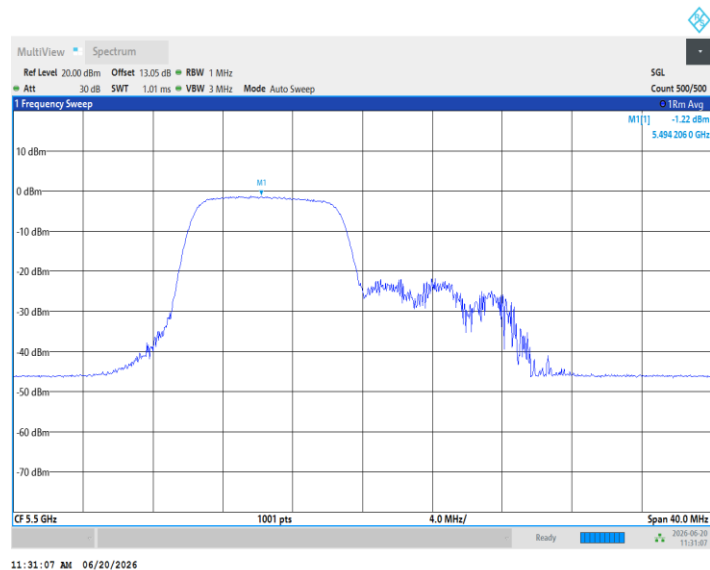
11AX20MIMO_Ant3_5500_106Tone_RU54
