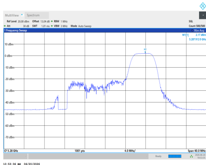
11AX20MIMO_Ant5_5280_106Tone_RU53
