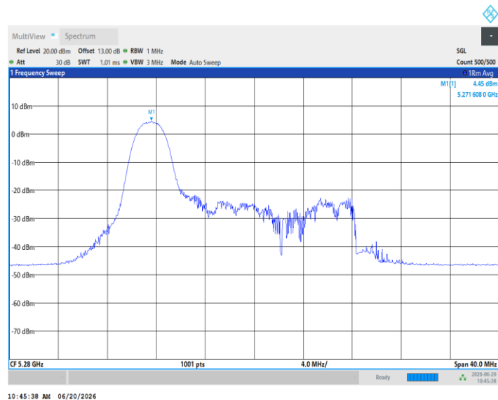
11AX20MIMO_Ant3_5280_26Tone_RU4
