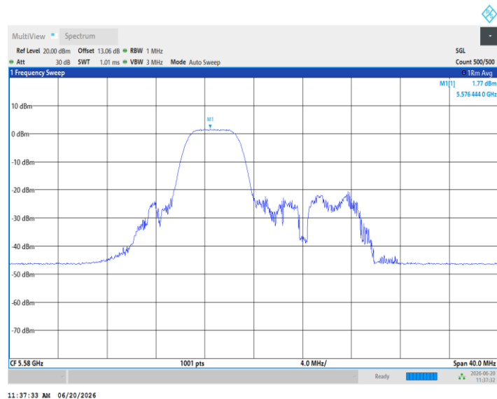
11AX20MIMO_Ant5_5580_52Tone_RU40
