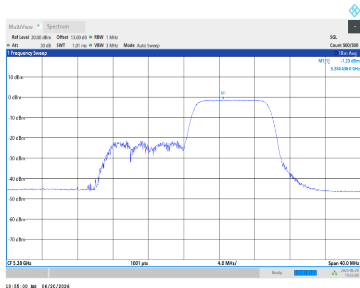
11AX20MIMO_Ant5_5280_26Tone_RU0
