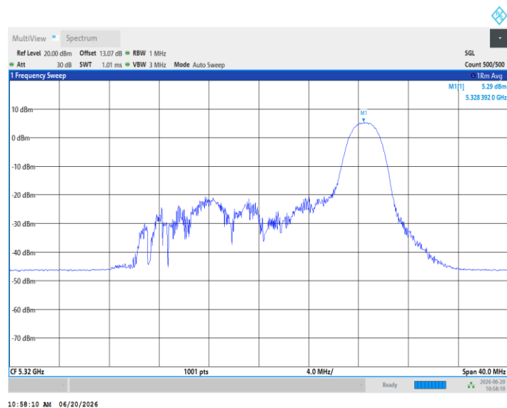
11AX20MIMO_Ant5_5320_52Tone_RU37
