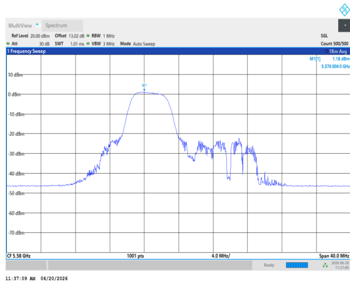
11AX20MIMO_Ant3_5580_52Tone_RU40
