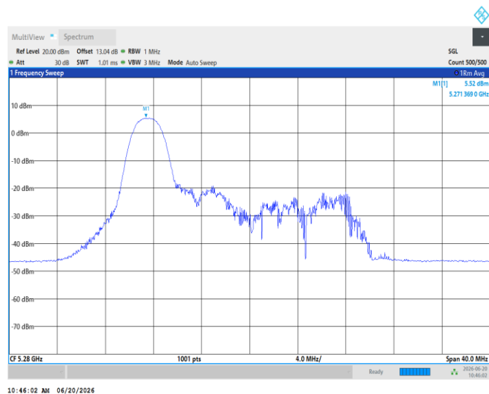
11AX20MIMO_Ant5_5280_26Tone_RU4
