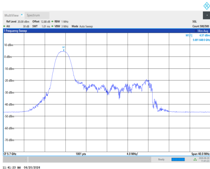
11AX20MIMO_Ant5_5700_26Tone_RU4
