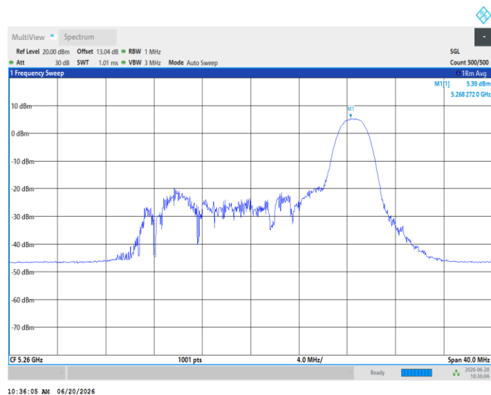
11AX20MIMO_Ant5_5260_52Tone_RU37
