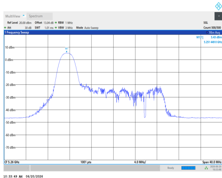
11AX20MIMO_Ant5_5260_26Tone_RU4
