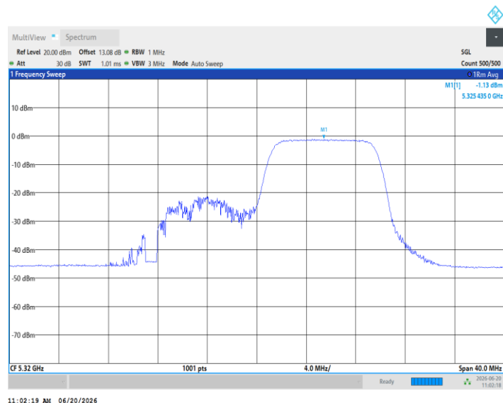
11AX20MIMO_Ant5_5320_26Tone_RU0
