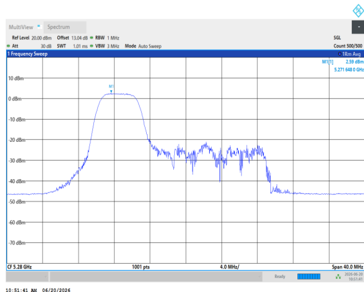
11AX20MIMO_Ant5_5280_52Tone_RU38
