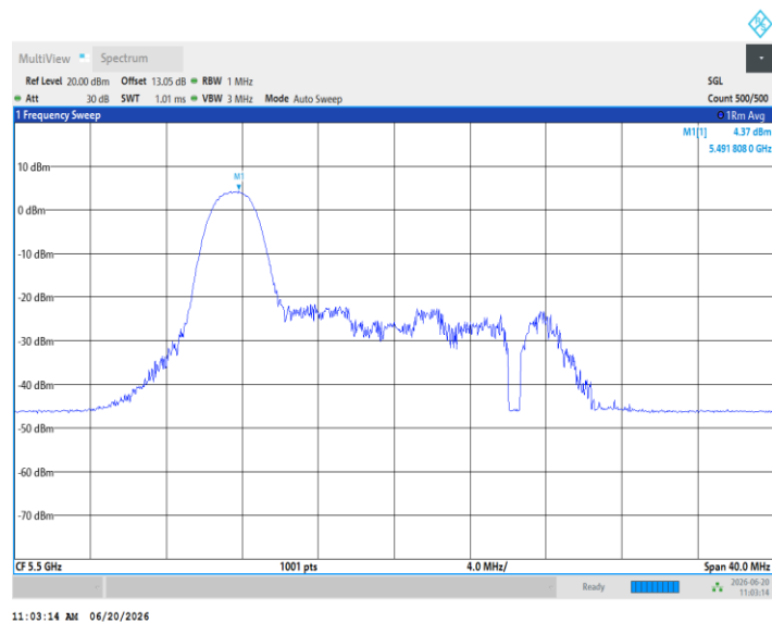
11AX20MIMO_Ant3_5500_26Tone_RU4
