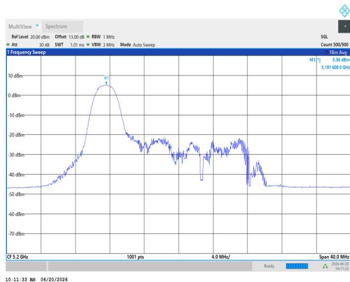
11AX20MIMO_Ant5_5200_26Tone_RU4
