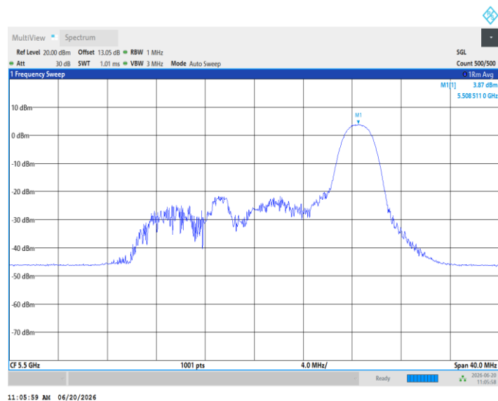
11AX20MIMO_Ant3_5500_52Tone_RU37
