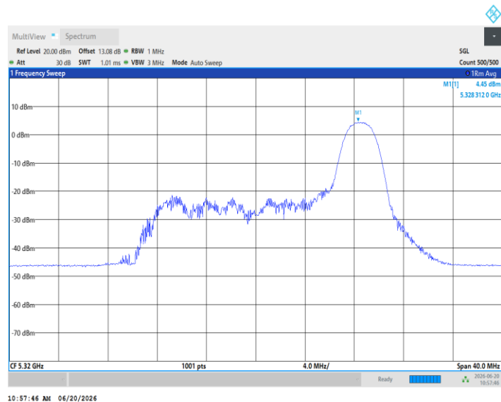
11AX20MIMO_Ant3_5320_52Tone_RU37
