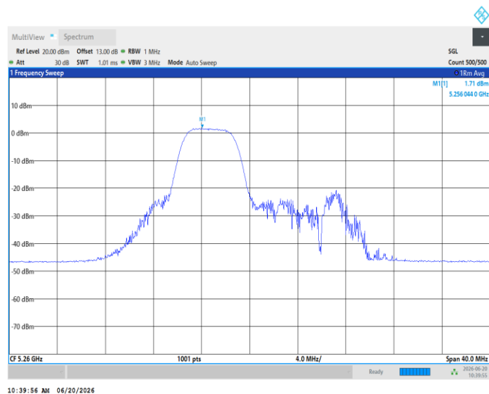
11AX20MIMO_Ant3_5260_52Tone_RU40
