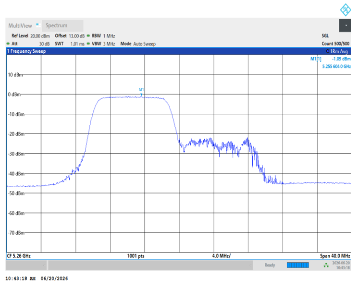
11AX20MIMO_Ant3_5260_106Tone_RU54
