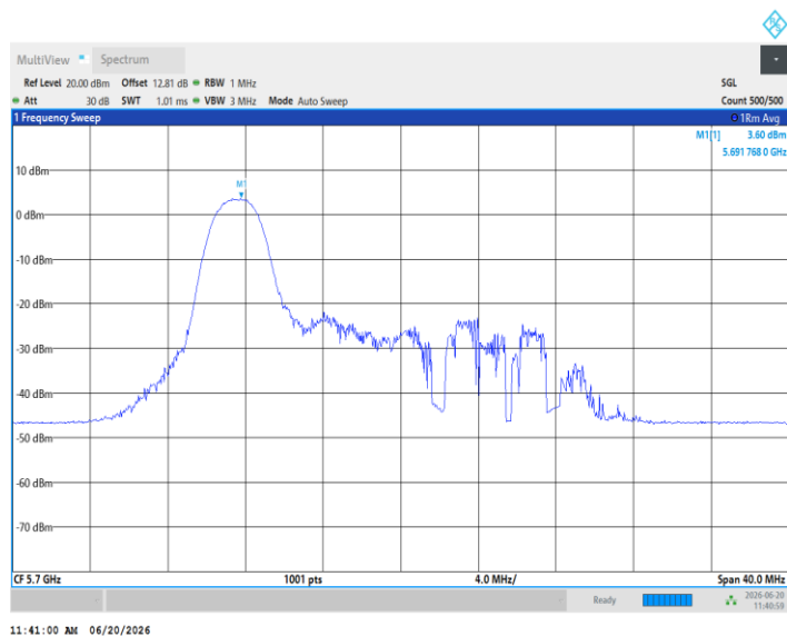
11AX20MIMO_Ant3_5700_26Tone_RU4
