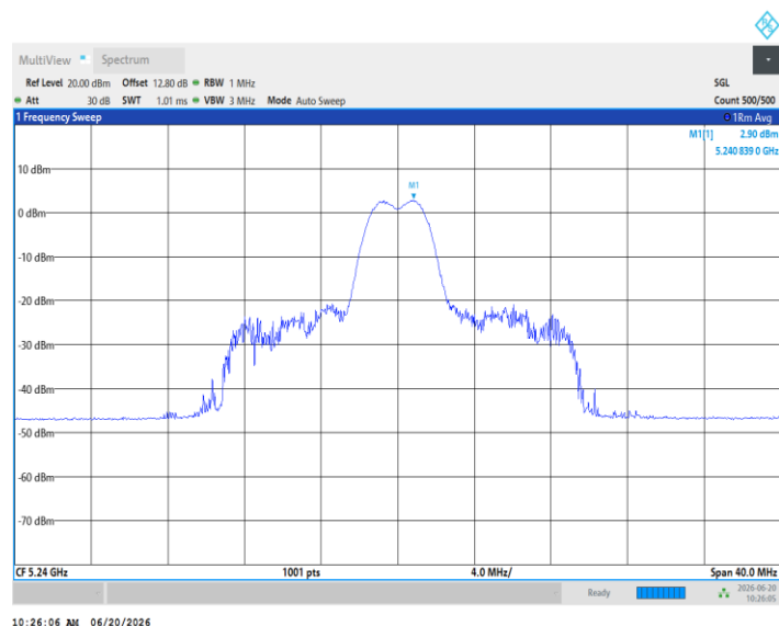
11AX20MIMO_Ant3_5240_26Tone_RU8
