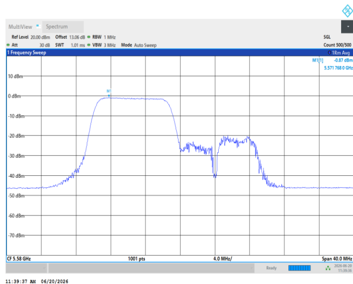
11AX20MIMO_Ant5_5580_106Tone_RU54
