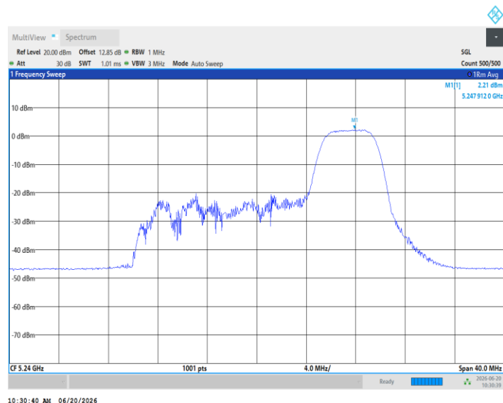
11AX20MIMO_Ant5_5240_106Tone_RU53
