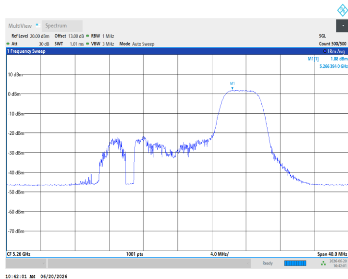
11AX20MIMO_Ant3_5260_106Tone_RU53
