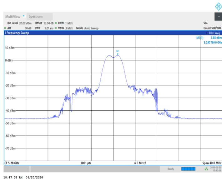
11AX20MIMO_Ant5_5280_26Tone_RU8
