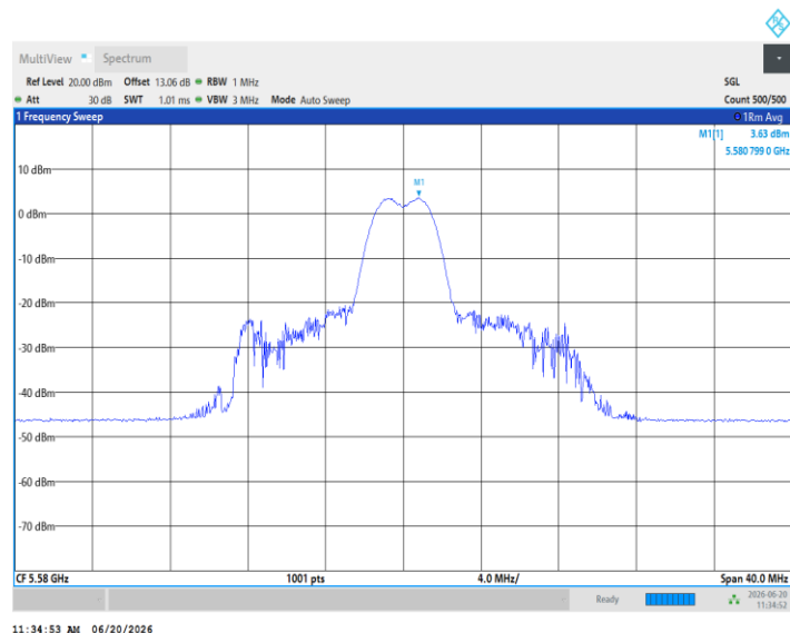
11AX20MIMO_Ant5_5580_26Tone_RU8
