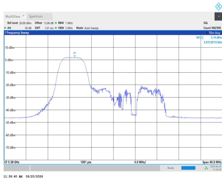
11AX20MIMO_Ant5_5580_52Tone_RU38
