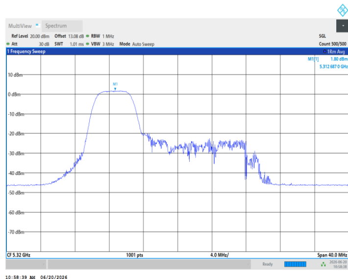
11AX20MIMO_Ant3_5320_52Tone_RU38
