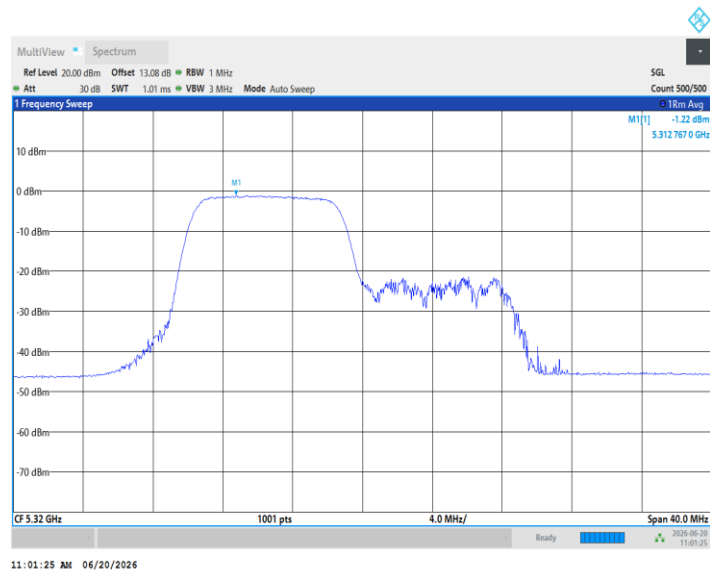
11AX20MIMO_Ant3_5320_106Tone_RU54
