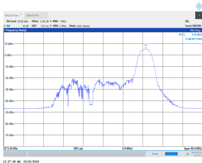
11AX20MIMO_Ant5_5240_52Tone_RU37
