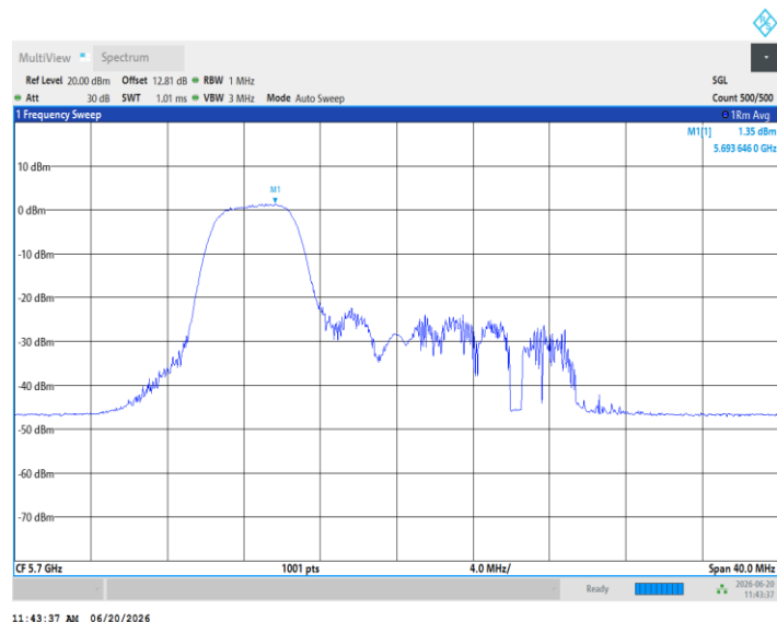
11AX20MIMO_Ant3_5700_52Tone_RU38
