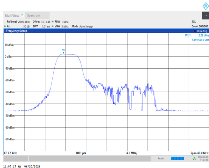
11AX20MIMO_Ant5_5500_52Tone_RU38
