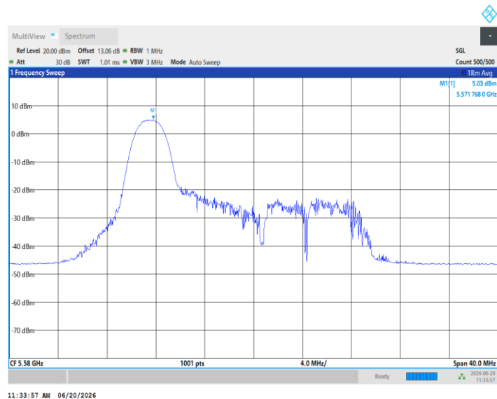
11AX20MIMO_Ant5_5580_26Tone_RU4
