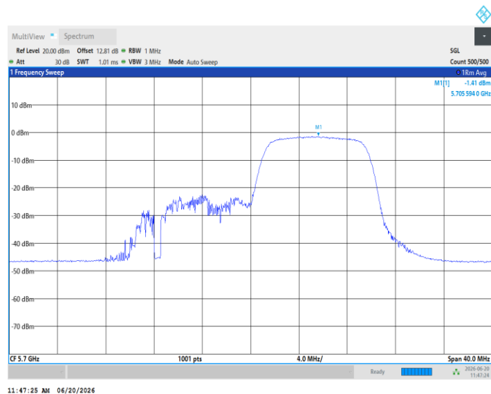
11AX20MIMO_Ant5_5700_26Tone_RU0
