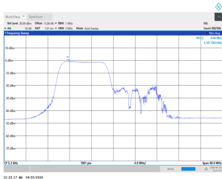
11AX20MIMO_Ant5_5200_106Tone_RU54
