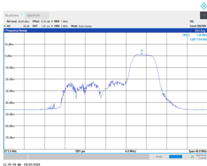
11AX20MIMO_Ant3_5500_106Tone_RU53
