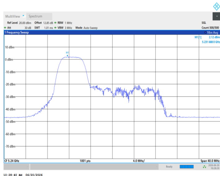
11AX20MIMO_Ant5_5240_52Tone_RU38
