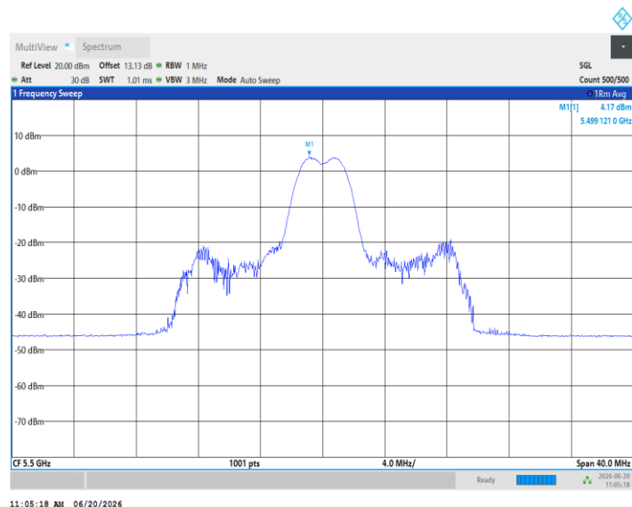
11AX20MIMO_Ant5_5500_26Tone_RU8
