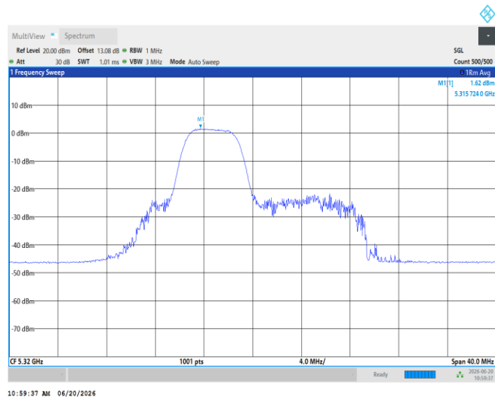
11AX20MIMO_Ant3_5320_52Tone_RU40
