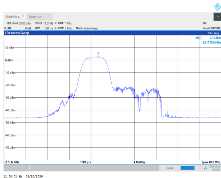
11AX20MIMO_Ant5_5320_52Tone_RU40
