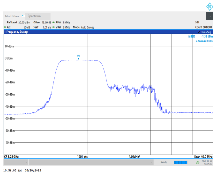
11AX20MIMO_Ant3_5280_106Tone_RU54
