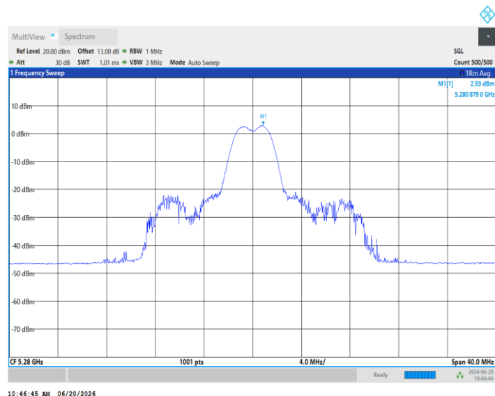
11AX20MIMO_Ant3_5280_26Tone_RU8
