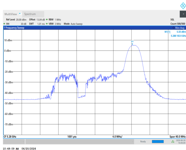
11AX20MIMO_Ant5_5280_52Tone_RU37
