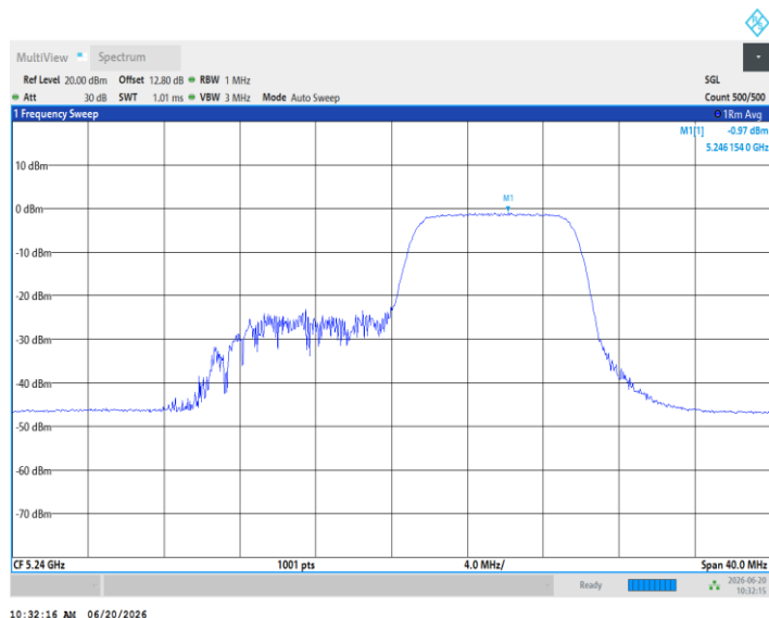
11AX20MIMO_Ant5_5240_26Tone_RU0
