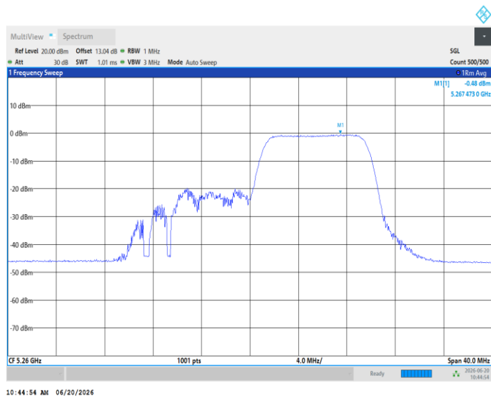
11AX20MIMO_Ant3_5280_26Tone_RU0
