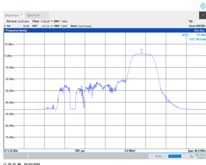
11AX20MIMO_Ant3_5320_106Tone_RU53
