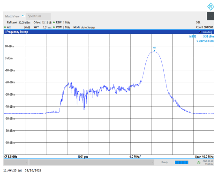
11AX20MIMO_Ant5_5500_52Tone_RU37
