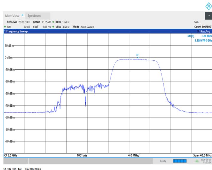
11AX20MIMO_Ant5_5500_26Tone_RU0
