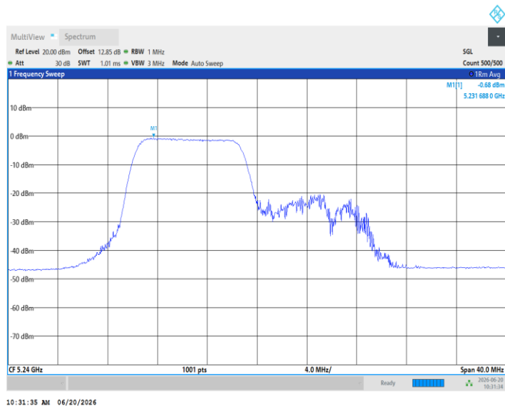
11AX20MIMO_Ant5_5240_106Tone_RU54
