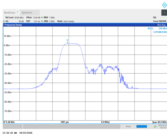
11AX20MIMO_Ant5_5280_52Tone_RU40
