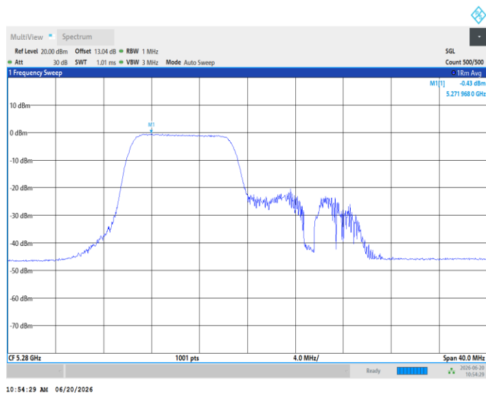
11AX20MIMO_Ant5_5280_106Tone_RU54
