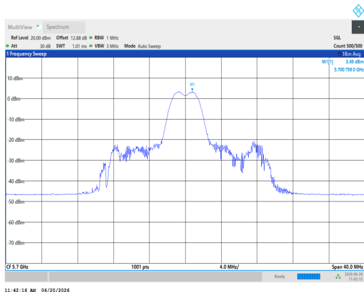
11AX20MIMO_Ant5_5700_26Tone_RU8
