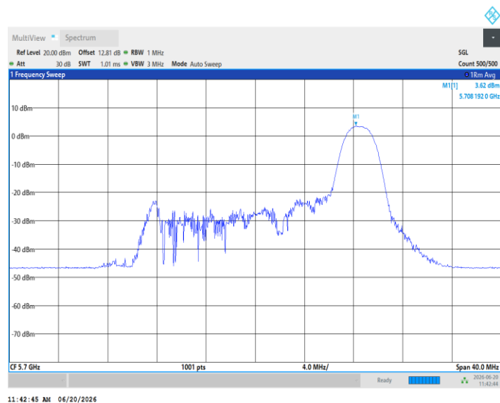
11AX20MIMO_Ant3_5700_52Tone_RU37
