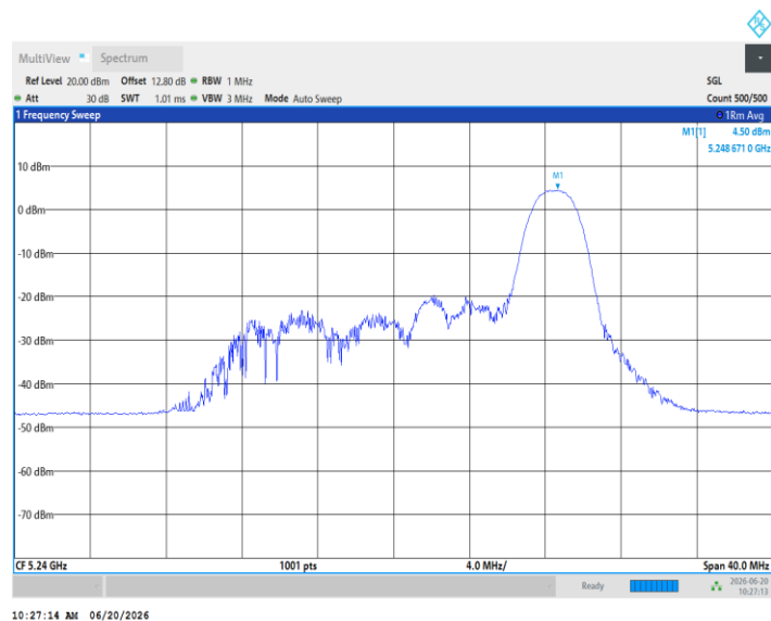
11AX20MIMO_Ant3_5240_52Tone_RU37
