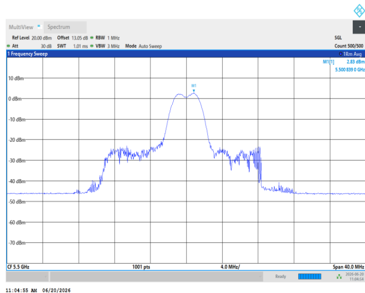
11AX20MIMO_Ant3_5500_26Tone_RU8
