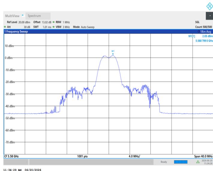
11AX20MIMO_Ant3_5580_26Tone_RU8
