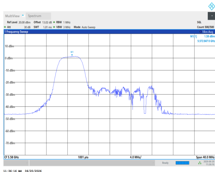
11AX20MIMO_Ant3_5580_52Tone_RU38
