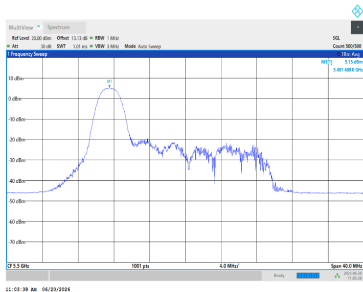
11AX20MIMO_Ant5_5500_26Tone_RU4
