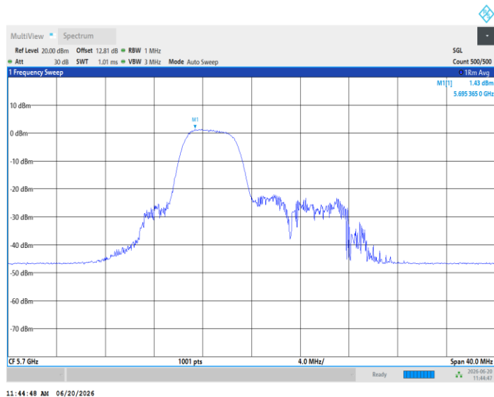
11AX20MIMO_Ant3_5700_52Tone_RU40
