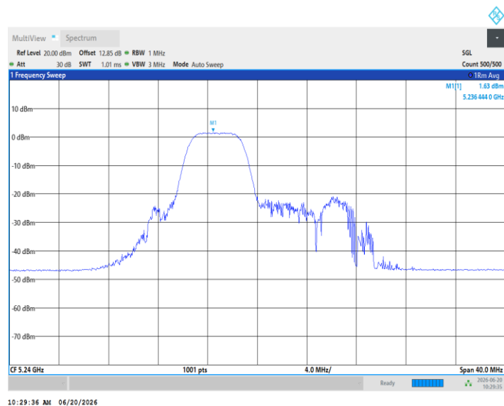
11AX20MIMO_Ant5_5240_52Tone_RU40
