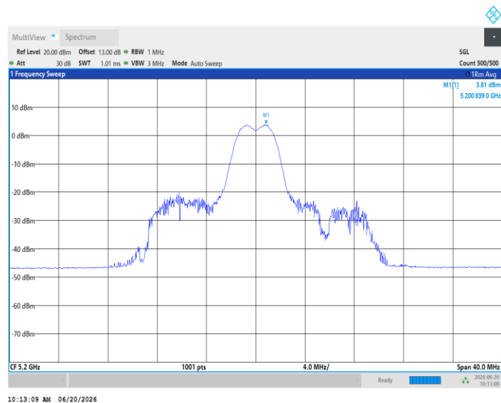
11AX20MIMO_Ant5_5200_26Tone_RU8
