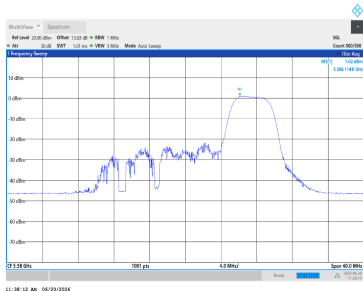
11AX20MIMO_Ant3_5580_106Tone_RU53
