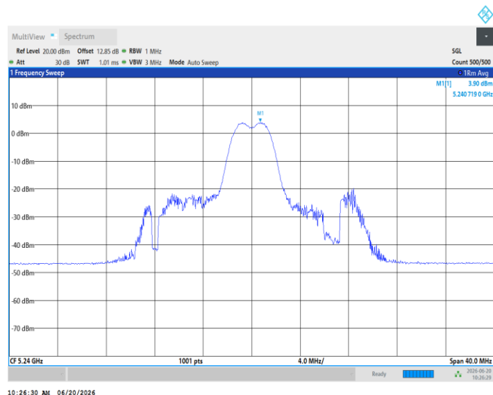
11AX20MIMO_Ant5_5240_26Tone_RU8
