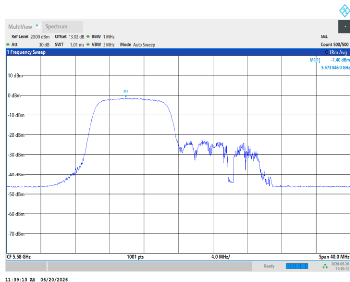
11AX20MIMO_Ant3_5580_106Tone_RU54
