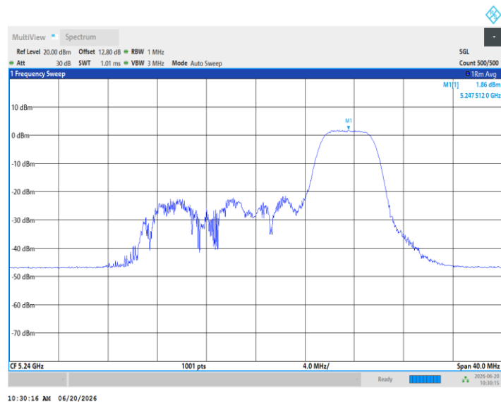
11AX20MIMO_Ant3_5240_106Tone_RU53
