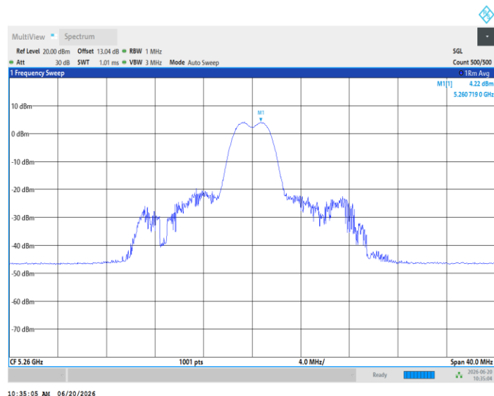
11AX20MIMO_Ant5_5260_26Tone_RU8
