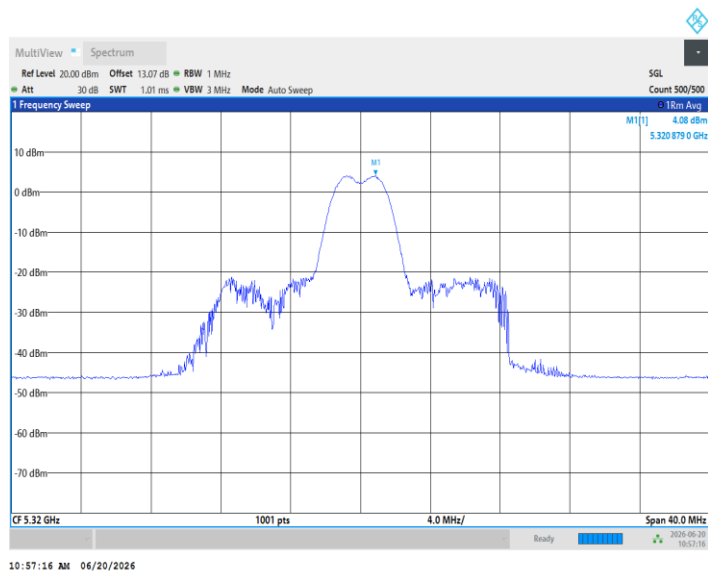
11AX20MIMO_Ant5_5320_26Tone_RU8
