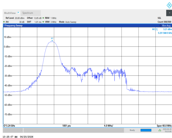
11AX20MIMO_Ant5_5240_26Tone_RU4
