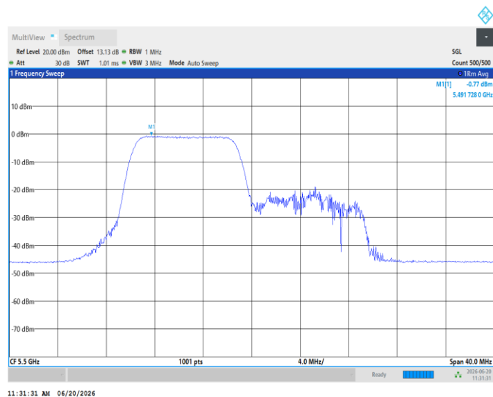
11AX20MIMO_Ant5_5500_106Tone_RU54
