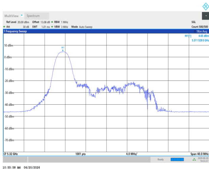
11AX20MIMO_Ant3_5320_26Tone_RU4
