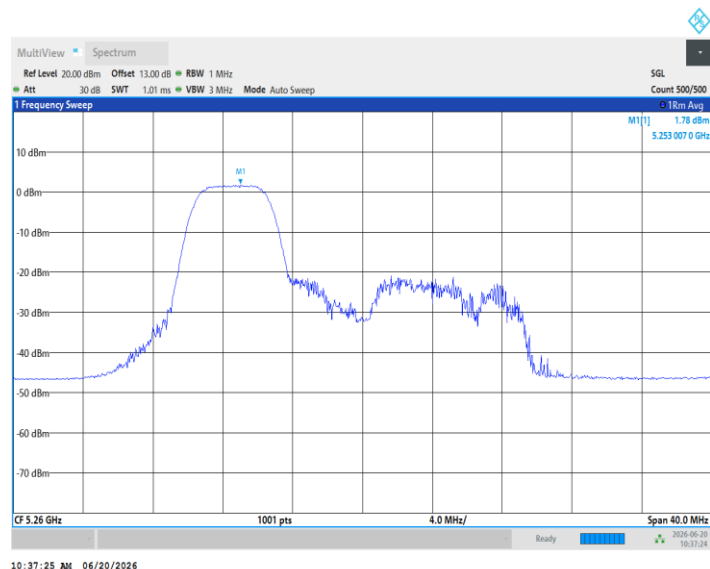
11AX20MIMO_Ant3_5260_52Tone_RU38
