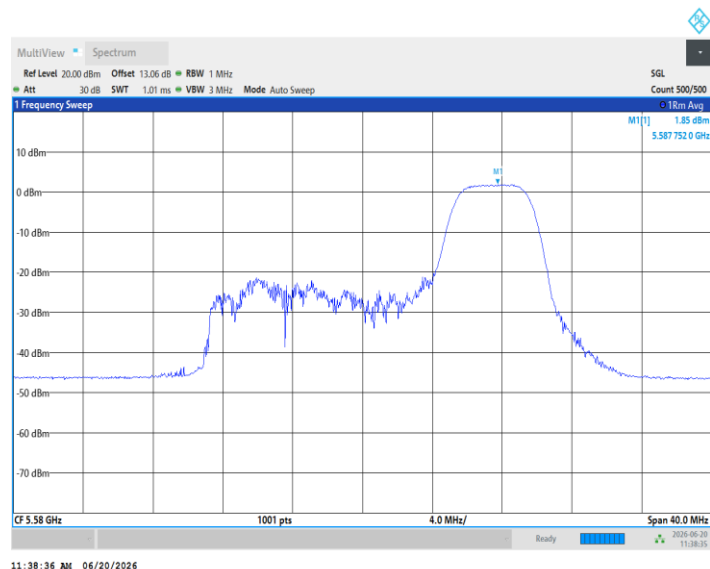
11AX20MIMO_Ant5_5580_106Tone_RU53
