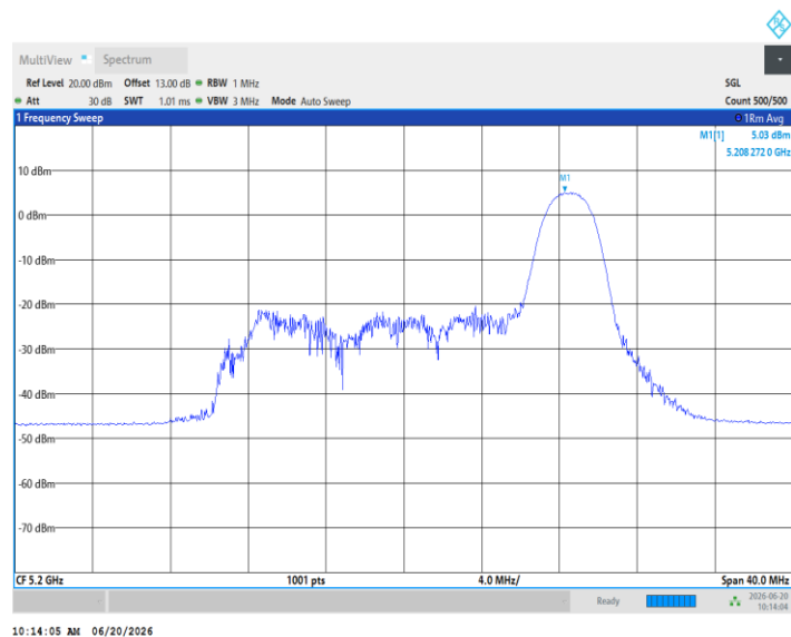
11AX20MIMO_Ant5_5200_52Tone_RU37
