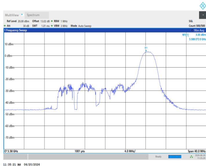
11AX20MIMO_Ant3_5580_52Tone_RU37
