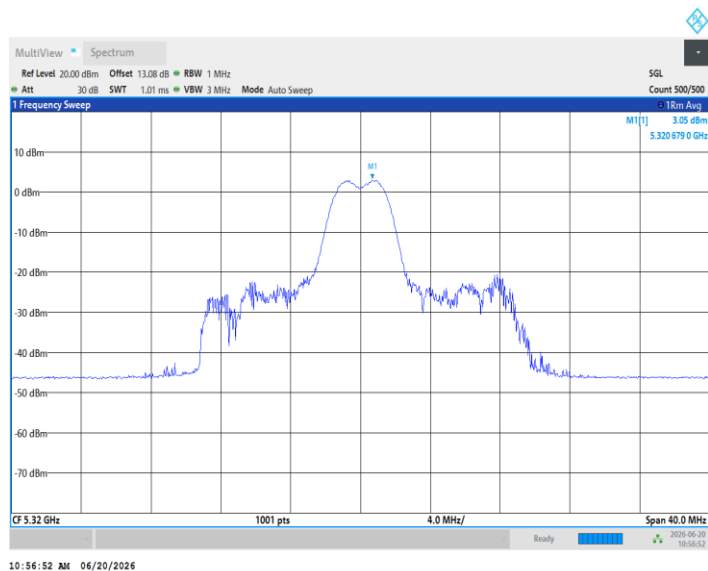
11AX20MIMO_Ant3_5320_26Tone_RU8
