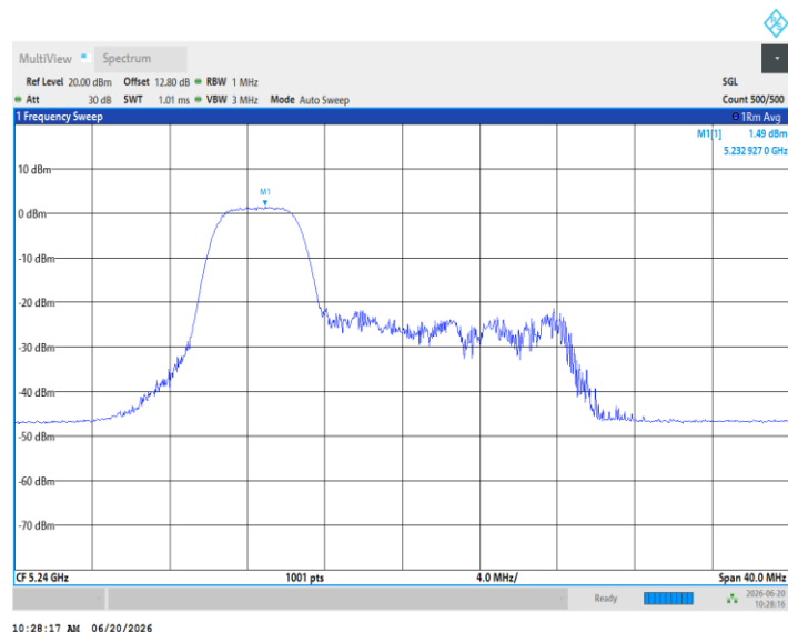
11AX20MIMO_Ant3_5240_52Tone_RU38
