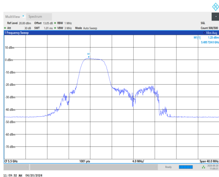
11AX20MIMO_Ant3_5500_52Tone_RU40
