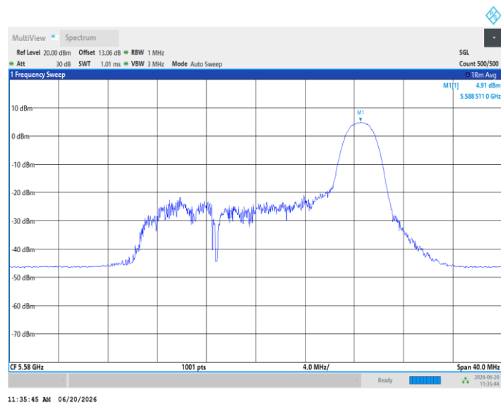
11AX20MIMO_Ant5_5580_52Tone_RU37
