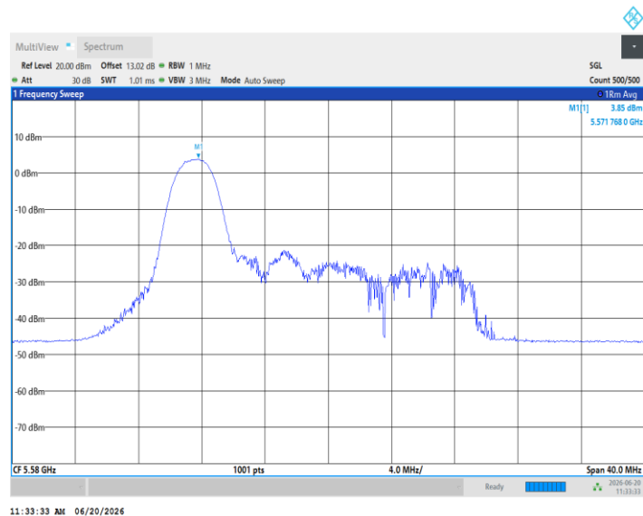
11AX20MIMO_Ant3_5580_26Tone_RU4
