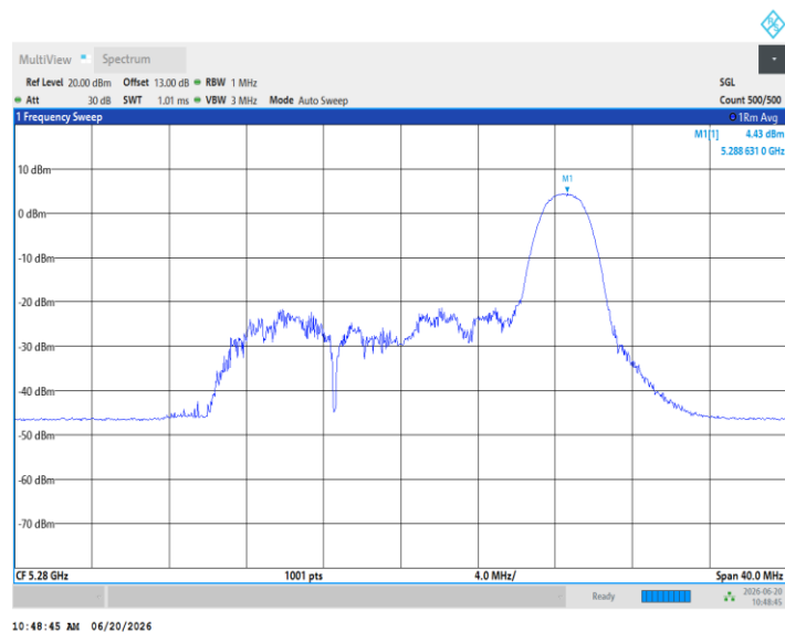
11AX20MIMO_Ant3_5280_52Tone_RU37
