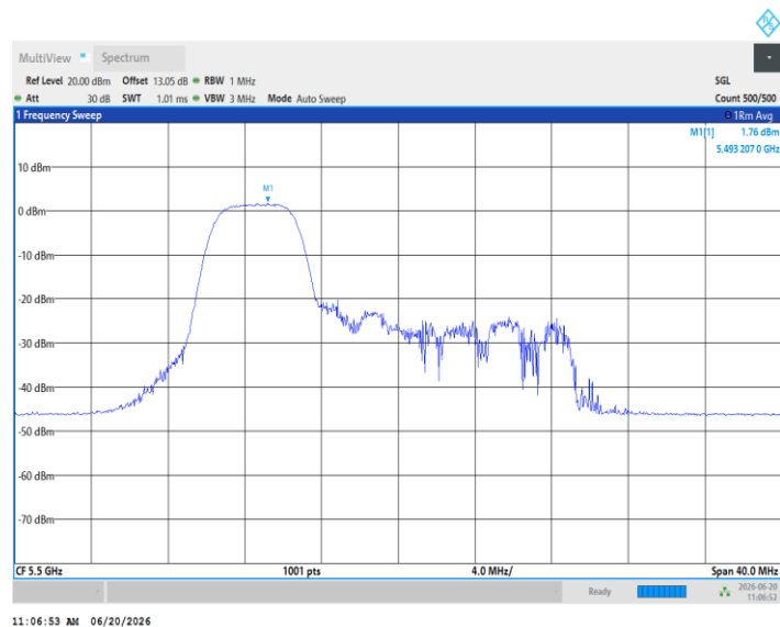
11AX20MIMO_Ant3_5500_52Tone_RU38
