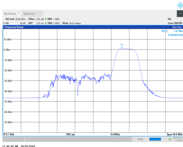
11AX20MIMO_Ant3_5700_106Tone_RU53
