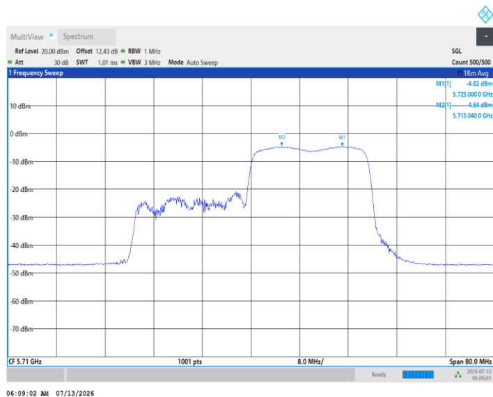
11AX40MIMO_Ant5_5710_UNII-2C_242Tone_RU61
