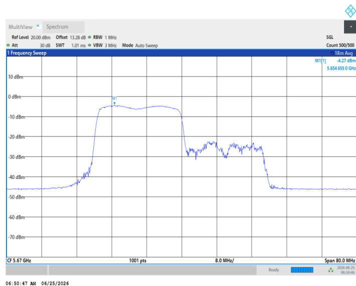
11AX40MIMO_Ant3_5670_242Tone_RU62
