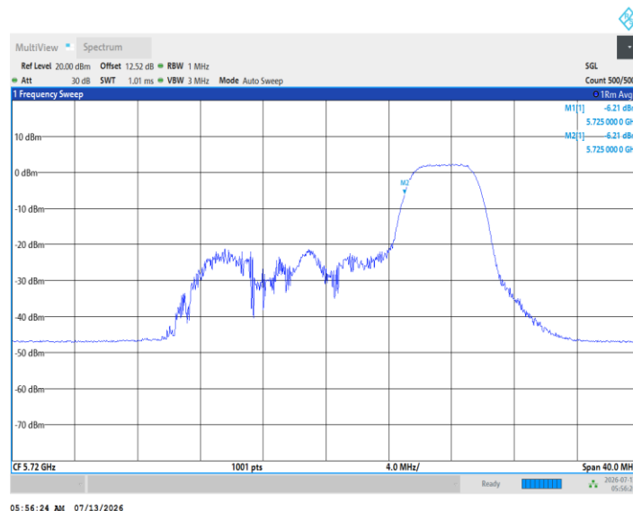
11AX20MIMO_Ant5_5720_UNII-2C_106Tone_RU53
