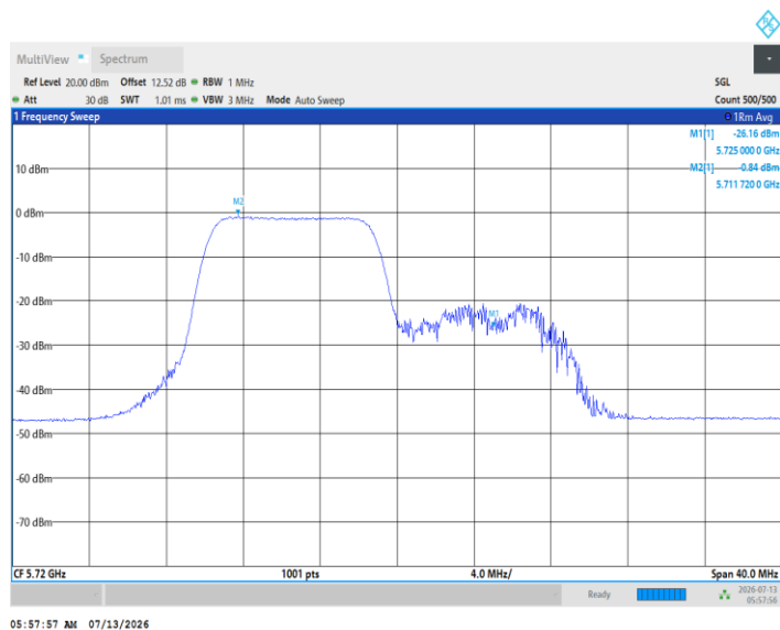
11AX20MIMO_Ant5_5720_UNII-2C_106Tone_RU54
