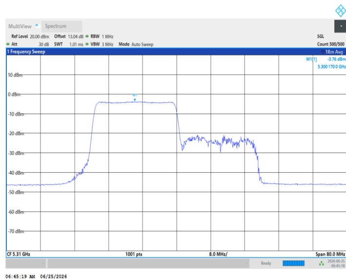
11AX40MIMO_Ant5_5310_242Tone_RU62
