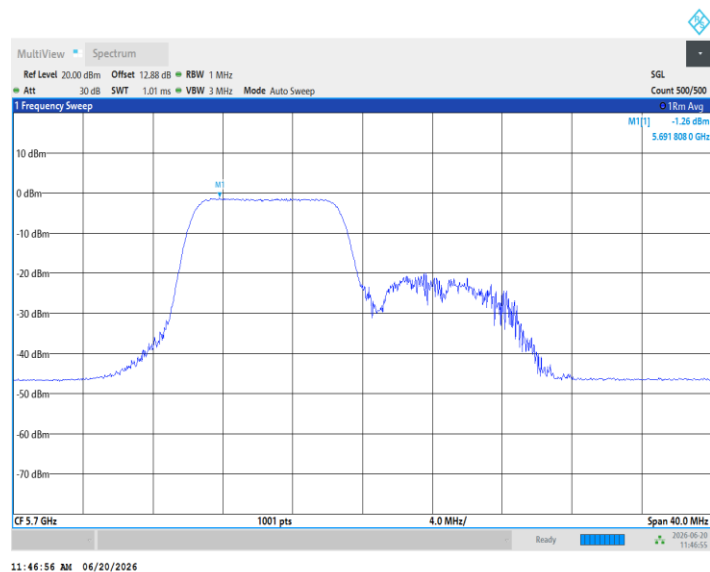
11AX20MIMO_Ant5_5700_106Tone_RU54
