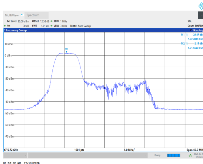
11AX20MIMO_Ant5_5720_UNII-2C_52Tone_RU38
