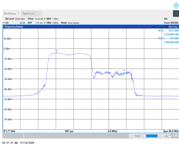
11AX40MIMO_Ant3_5710_UNII-2C_242Tone_RU62
