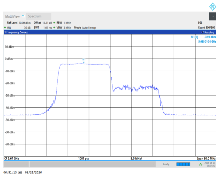
11AX40MIMO_Ant5_5670_242Tone_RU62
