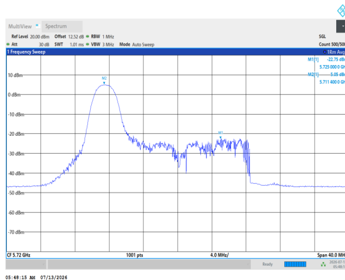
11AX20MIMO_Ant5_5720_UNII-2C_26Tone_RU4
