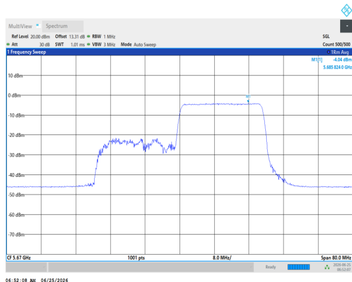
11AX40MIMO_Ant3_5710_UNII-2C_242Tone_RU61
