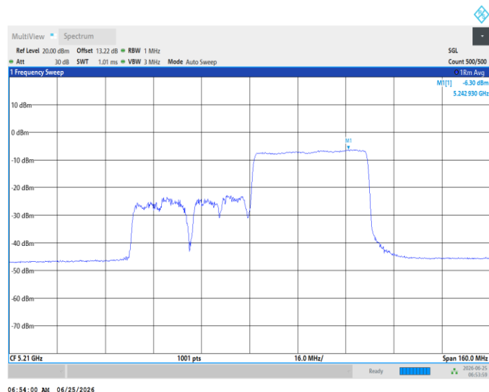
11AX80MIMO_Ant5_5210_484Tone_RU65
