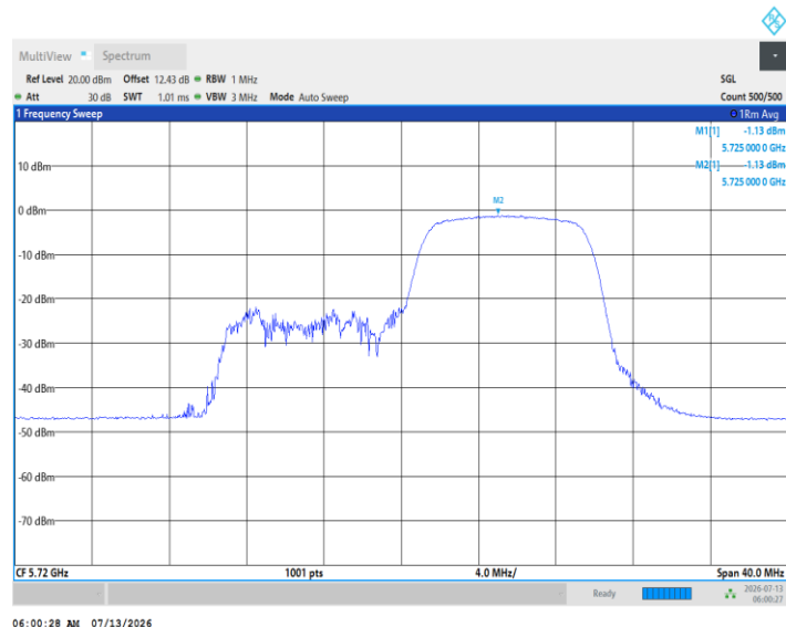
11AX20MIMO_Ant5_5720_UNII-2C_26Tone_RU0
