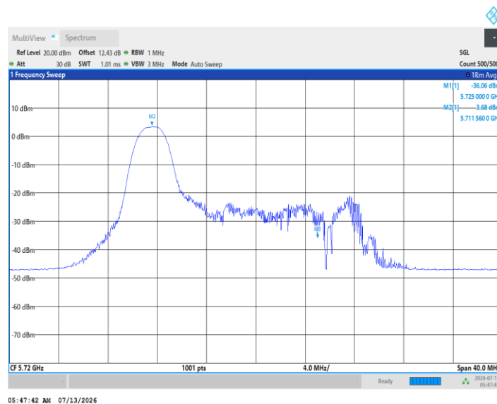
11AX20MIMO_Ant3_5720_UNII-2C_26Tone_RU4
