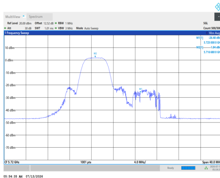
11AX20MIMO_Ant5_5720_UNII-2C_52Tone_RU40
