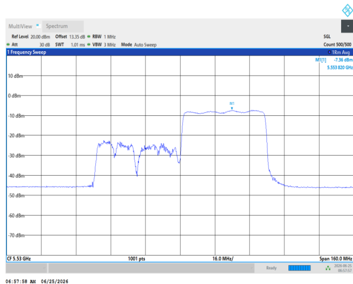
11AX80MIMO_Ant5_5530_484Tone_RU65
