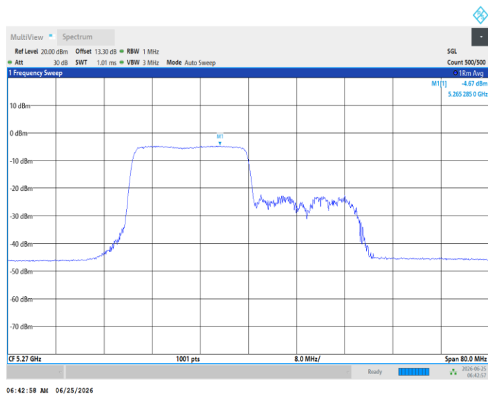
11AX40MIMO_Ant3_5270_242Tone_RU62
