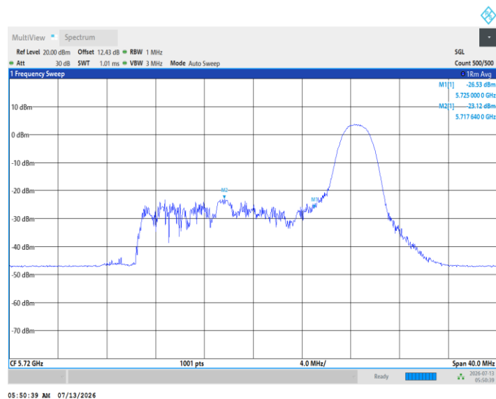
11AX20MIMO_Ant3_5720_UNII-2C_52Tone_RU37
