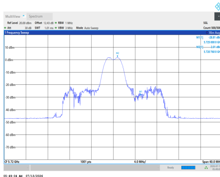
11AX20MIMO_Ant3_5720_UNII-2C_26Tone_RU8
