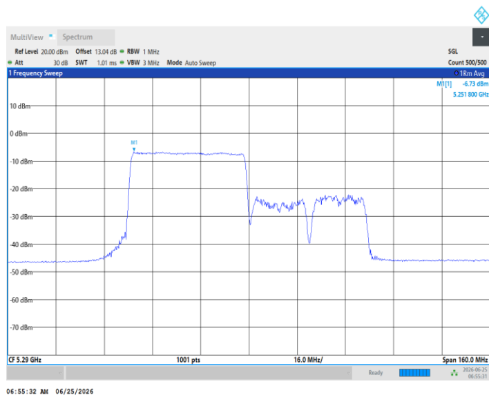
11AX80MIMO_Ant5_5290_484Tone_RU66
