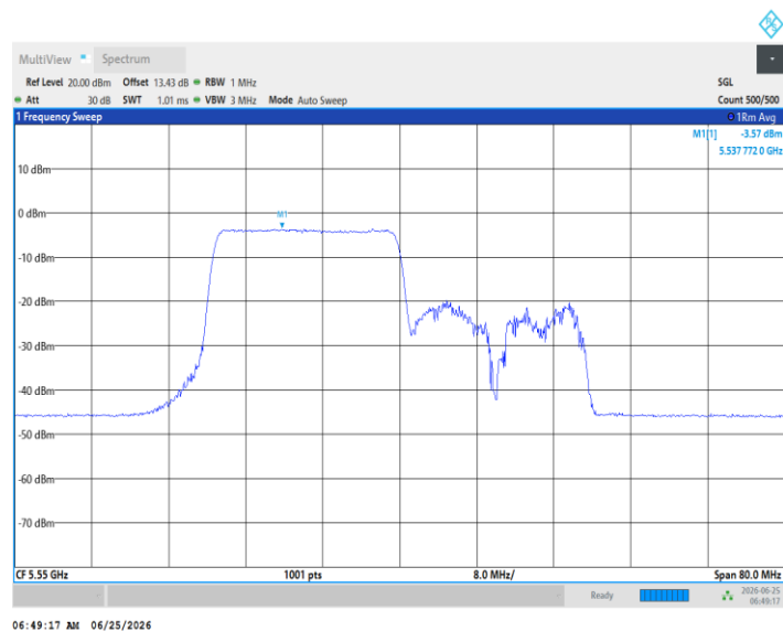
11AX40MIMO_Ant5_5550_242Tone_RU62
