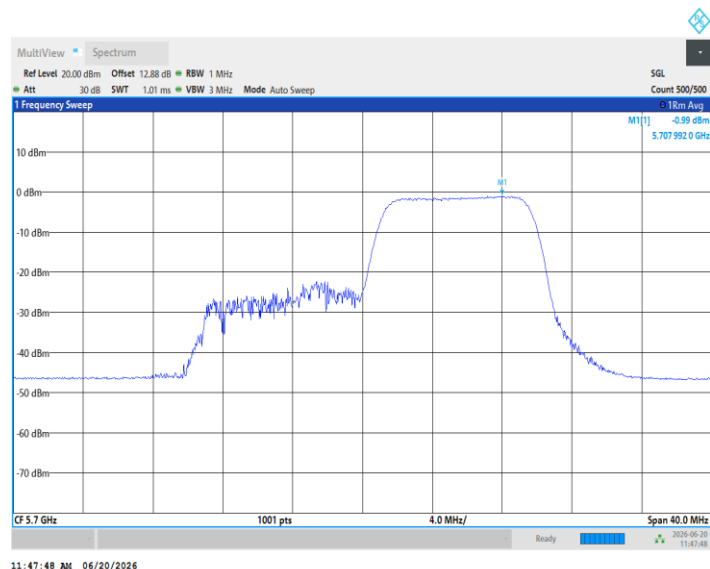
11AX20MIMO_Ant3_5720_UNII-2C_26Tone_RU0
