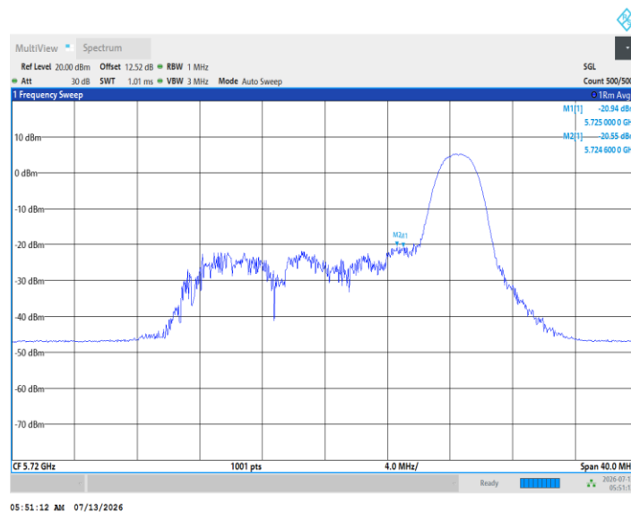
11AX20MIMO_Ant5_5720_UNII-2C_52Tone_RU37
