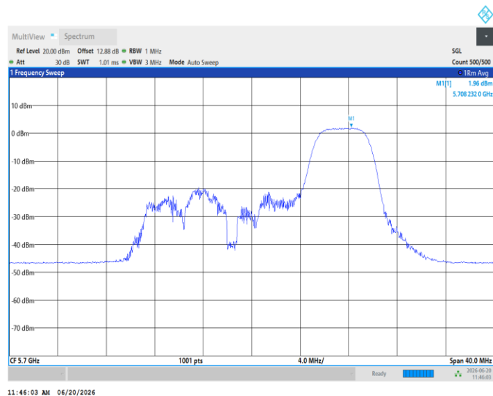
11AX20MIMO_Ant5_5700_106Tone_RU53
