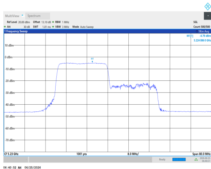
11AX40MIMO_Ant3_5230_242Tone_RU62
