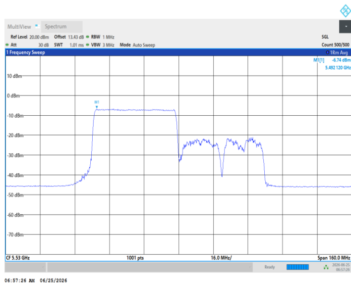
11AX80MIMO_Ant5_5530_484Tone_RU66
