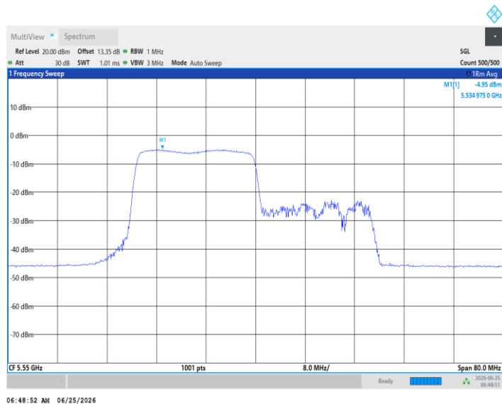
11AX40MIMO_Ant3_5550_242Tone_RU62
