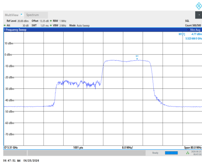
11AX40MIMO_Ant5_5510_242Tone_RU61
