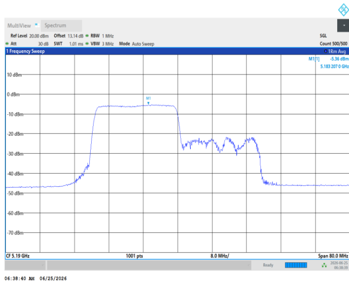
11AX40MIMO_Ant3_5190_242Tone_RU62
