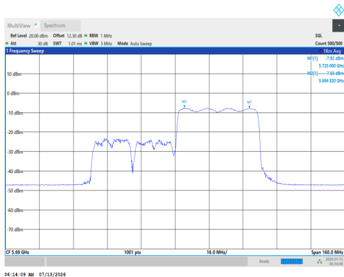
11AX80MIMO_Ant5_5690_UNII-2C_484Tone_RU65
