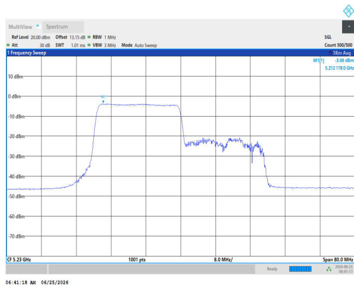
11AX40MIMO_Ant5_5230_242Tone_RU62
