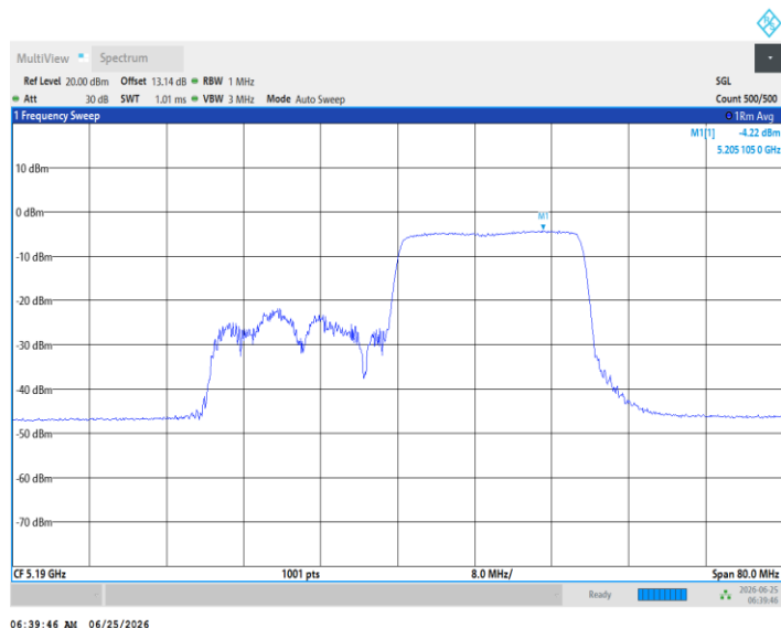
11AX40MIMO_Ant5_5190_242Tone_RU61
