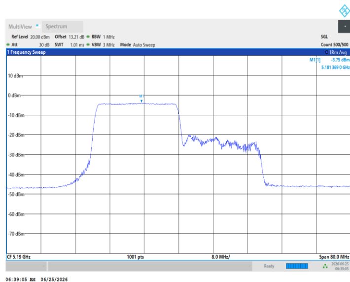
11AX40MIMO_Ant5_5190_242Tone_RU62
