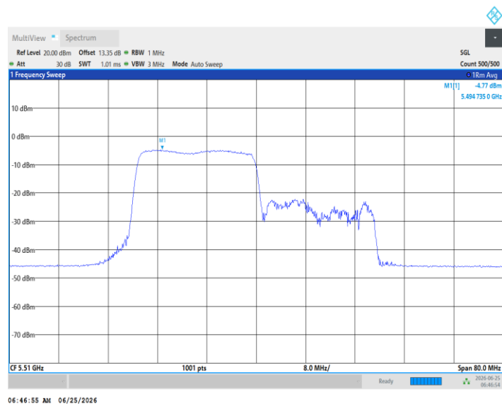
11AX40MIMO_Ant3_5510_242Tone_RU62
