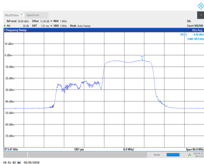
11AX40MIMO_Ant5_5670_242Tone_RU61
