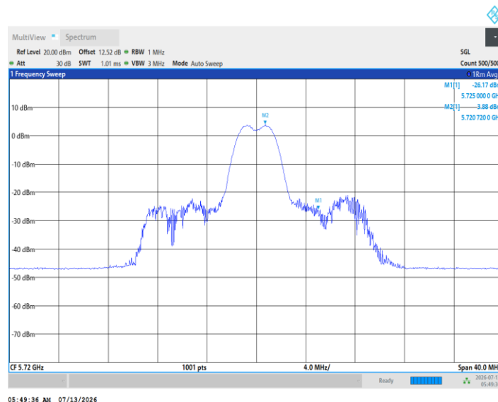
11AX20MIMO_Ant5_5720_UNII-2C_26Tone_RU8
