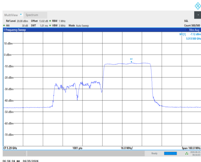
11AX80MIMO_Ant5_5290_484Tone_RU65
