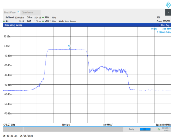
11AX40MIMO_Ant5_5270_242Tone_RU62
