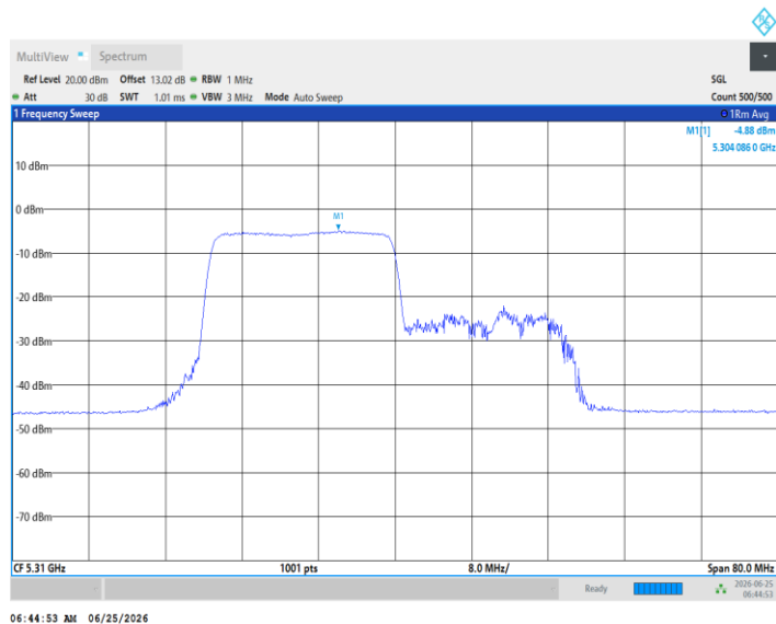
11AX40MIMO_Ant3_5310_242Tone_RU62
