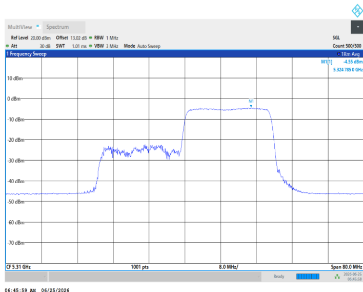
11AX40MIMO_Ant5_5310_242Tone_RU61
