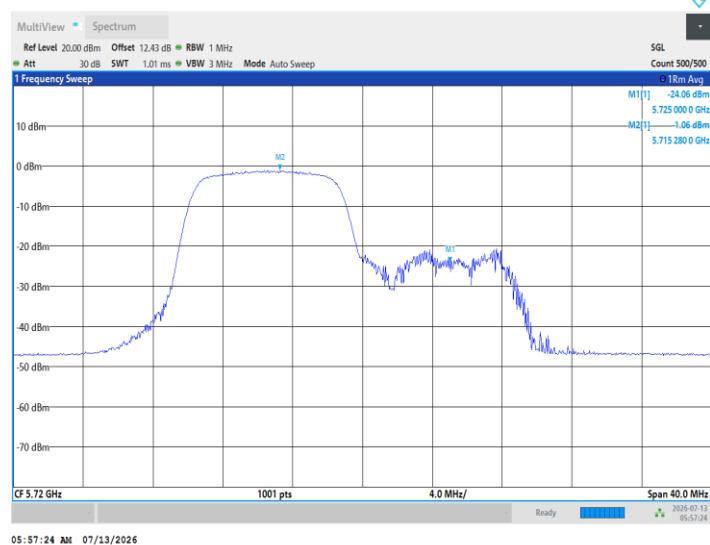
11AX20MIMO_Ant3_5720_UNII-2C_106Tone_RU54
