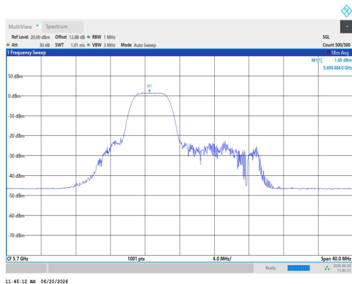
11AX20MIMO_Ant5_5700_52Tone_RU40
