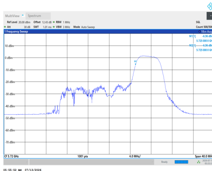
11AX20MIMO_Ant3_5720_UNII-2C_106Tone_RU53
