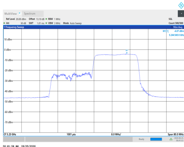
11AX40MIMO_Ant5_5230_242Tone_RU61
