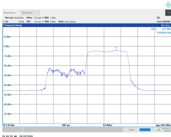
11AX40MIMO_Ant5_5550_242Tone_RU61
