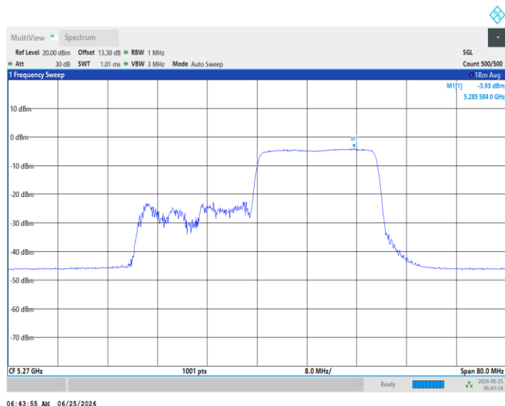
11AX40MIMO_Ant5_5270_242Tone_RU61
