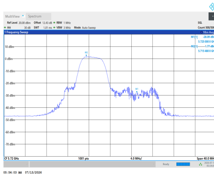
11AX20MIMO_Ant3_5720_UNII-2C_52Tone_RU40
