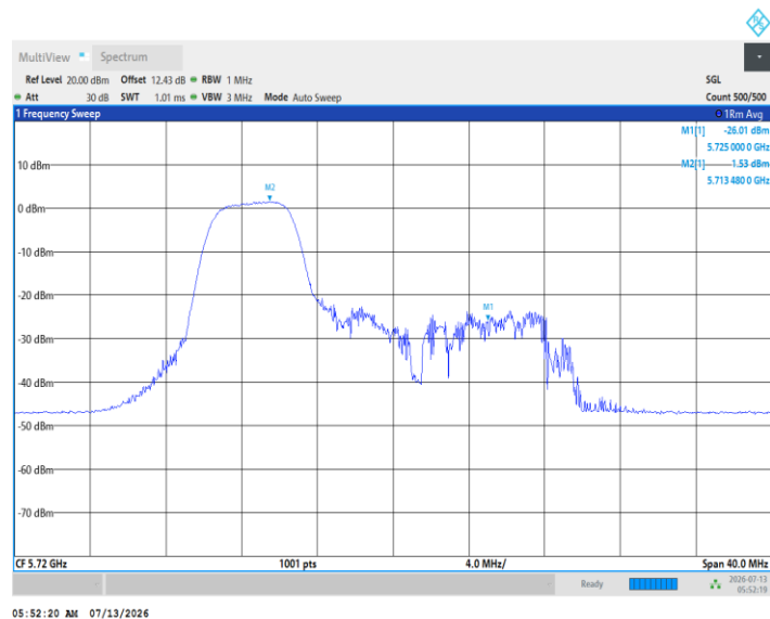
11AX20MIMO_Ant3_5720_UNII-2C_52Tone_RU38
