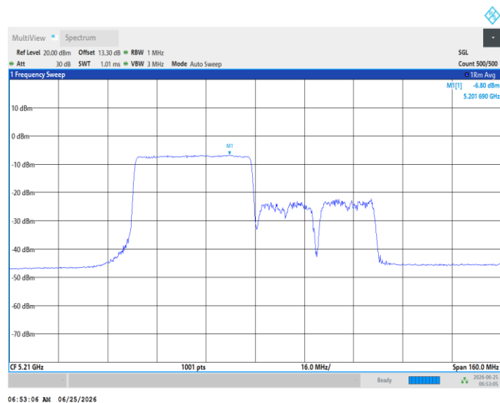
11AX80MIMO_Ant5_5210_484Tone_RU66
