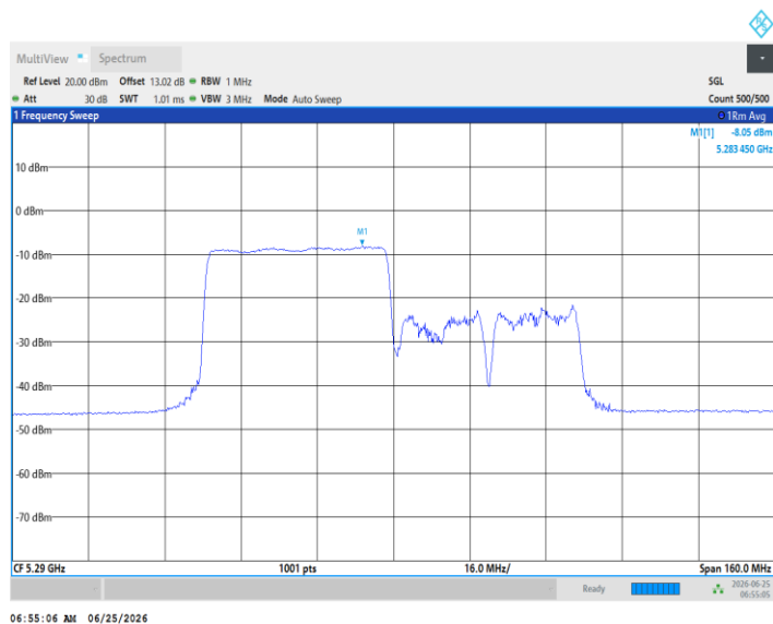
11AX80MIMO_Ant3_5290_484Tone_RU66
