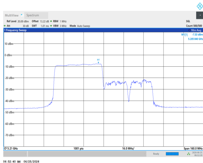
11AX80MIMO_Ant3_5210_484Tone_RU66
