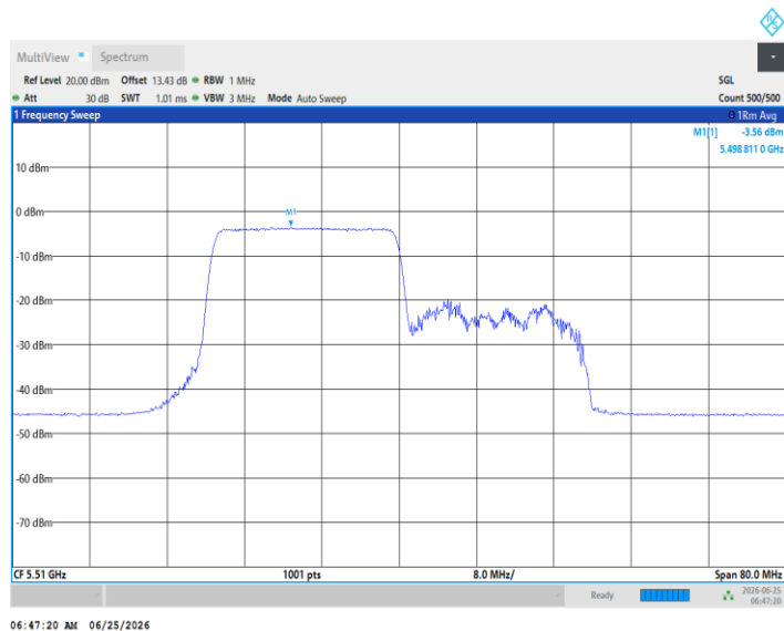
11AX40MIMO_Ant5_5510_242Tone_RU62
