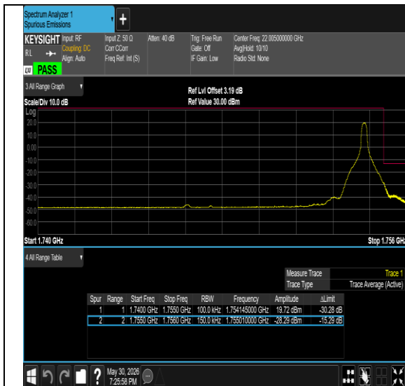
Band4-20MHz-QPSK-20050-1RB#0-PASS
