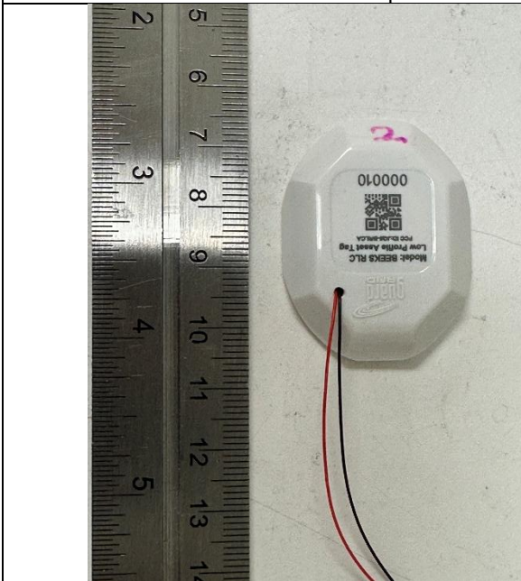
BVBRLC-LP-AT -Top
