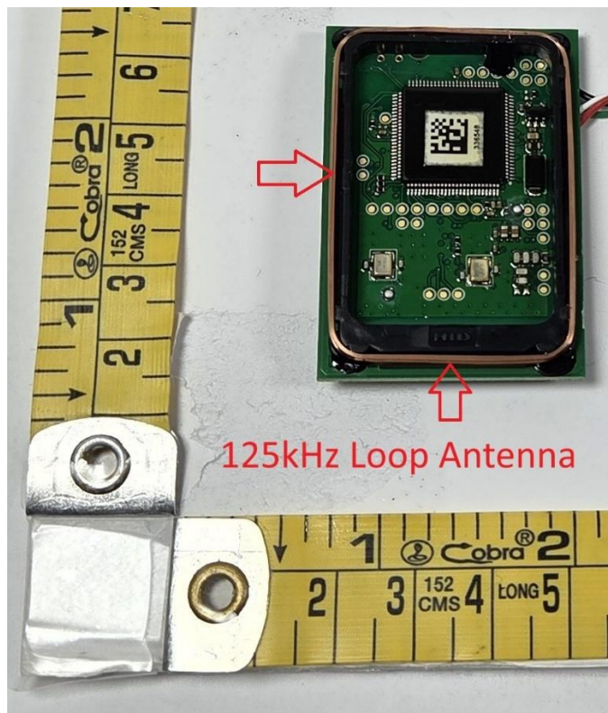
OMNIKEY 5127CK MINI Encoder_LF Antenna Location_Bottom Side
