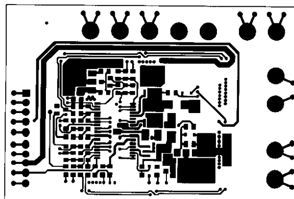
Copper Layer 4
