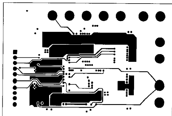
Copper Layer 3
