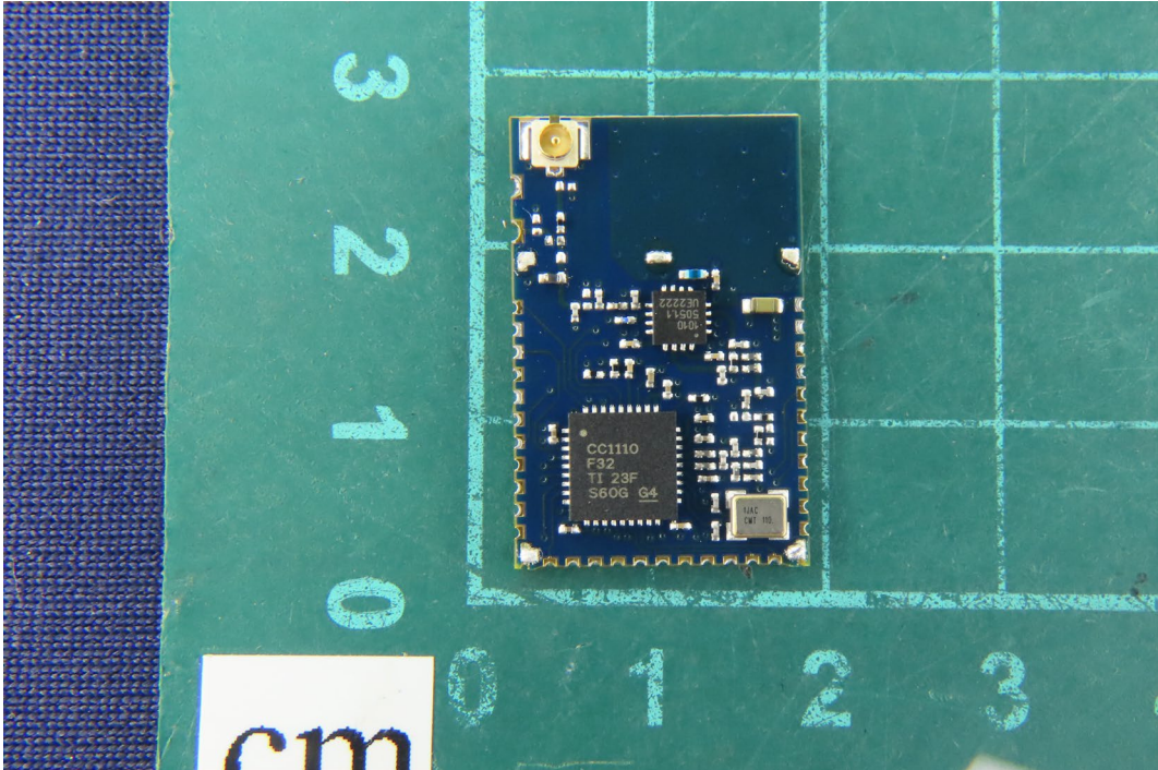
(26) EUT Photo_RFID Module
