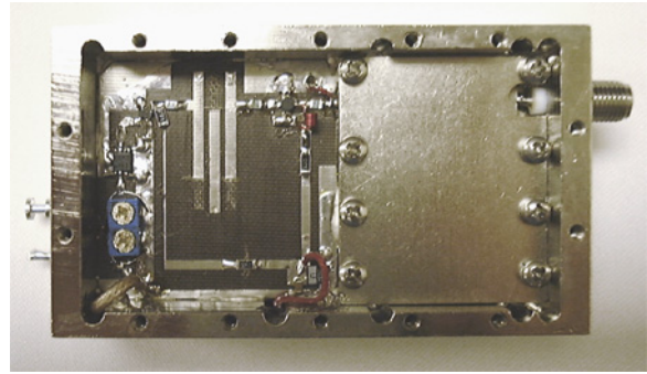
P/N: 87225-013 (Back)
