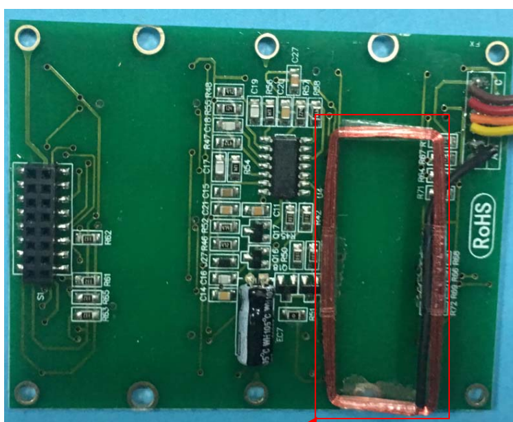
Antenna
