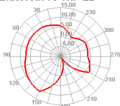
Bluetooth 78 TRP E2
