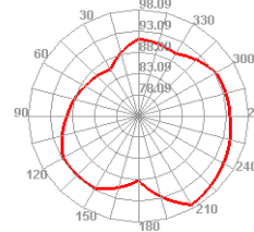
Bluetooth 39 TIS E1
