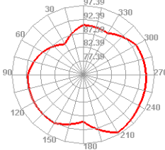
Bluetooth 0 TIS E1
