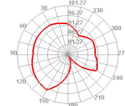
Bluetooth 78 TIS E2
