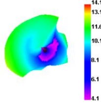
Bluetooth 39 TRP E1
