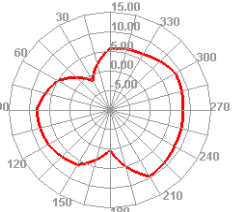
Bluetooth 78 TRP E1
