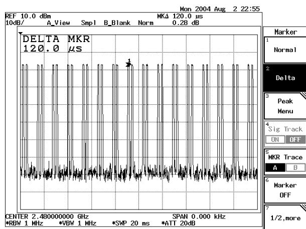
CH 78 2480MHz
