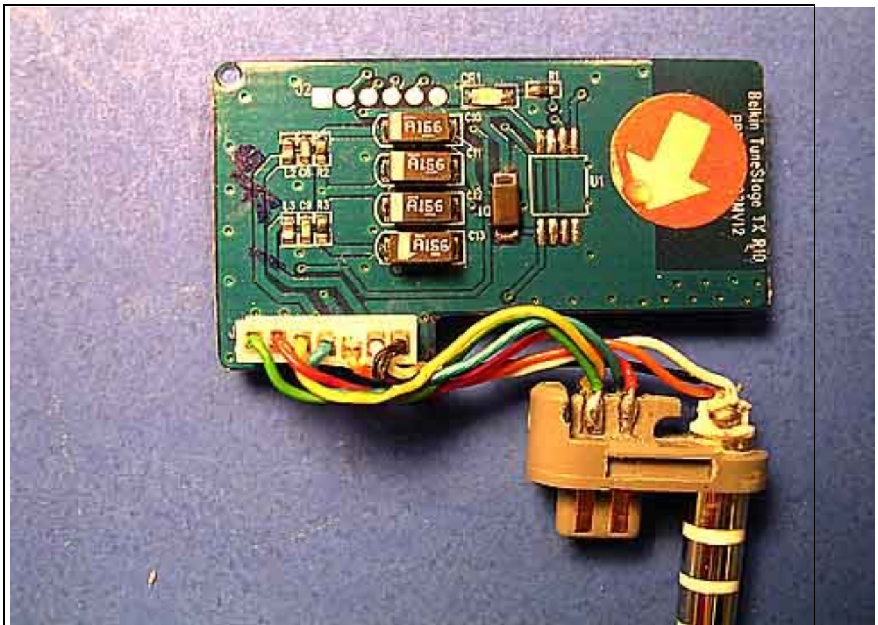
TX PCB Bottom
