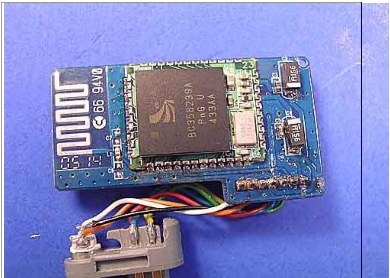
TX PCB Top 1
