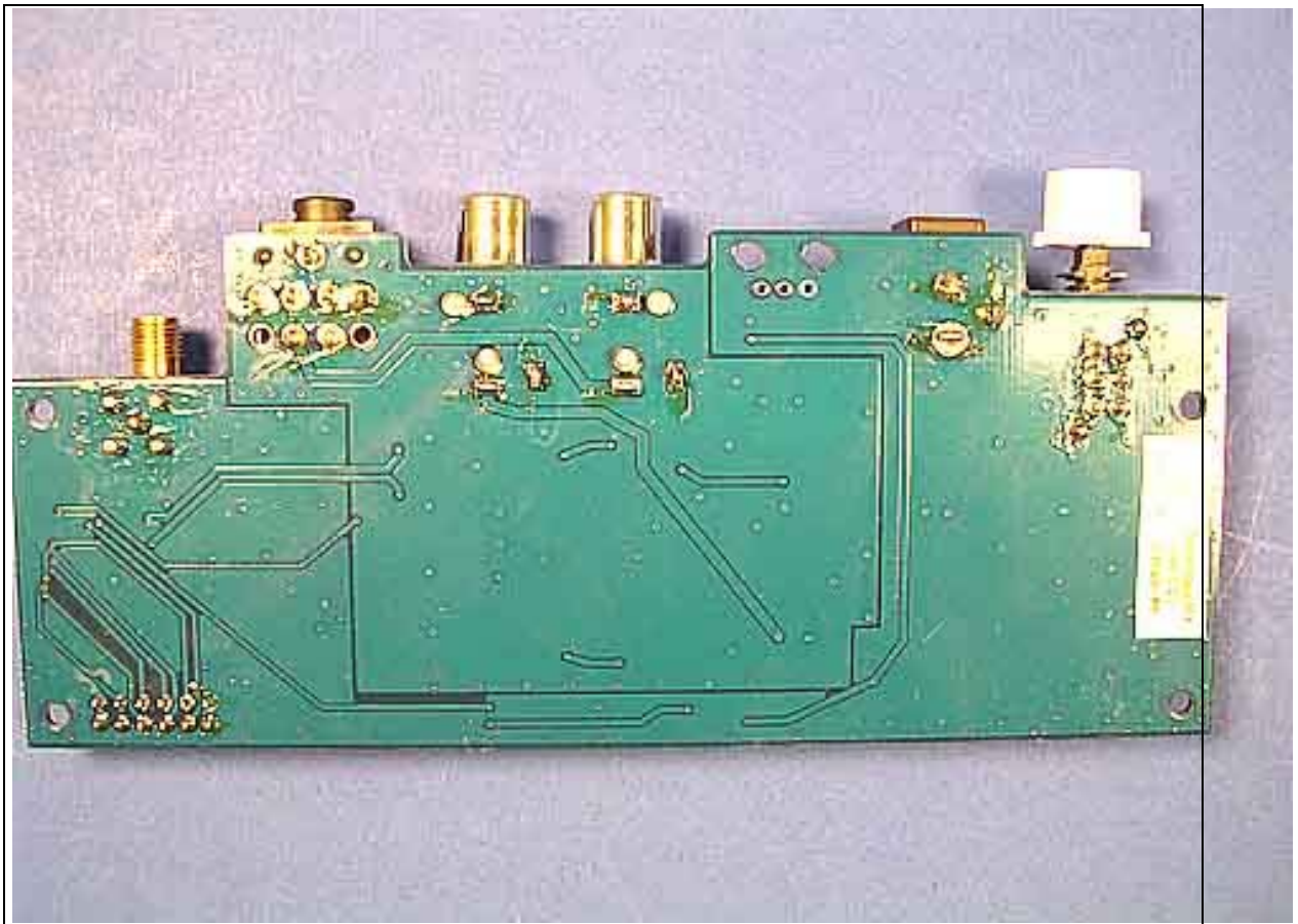
RX PCB Bottom
