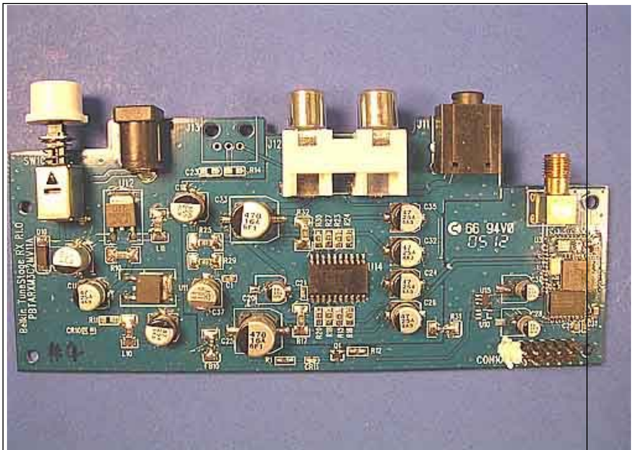
RX PCB Top
