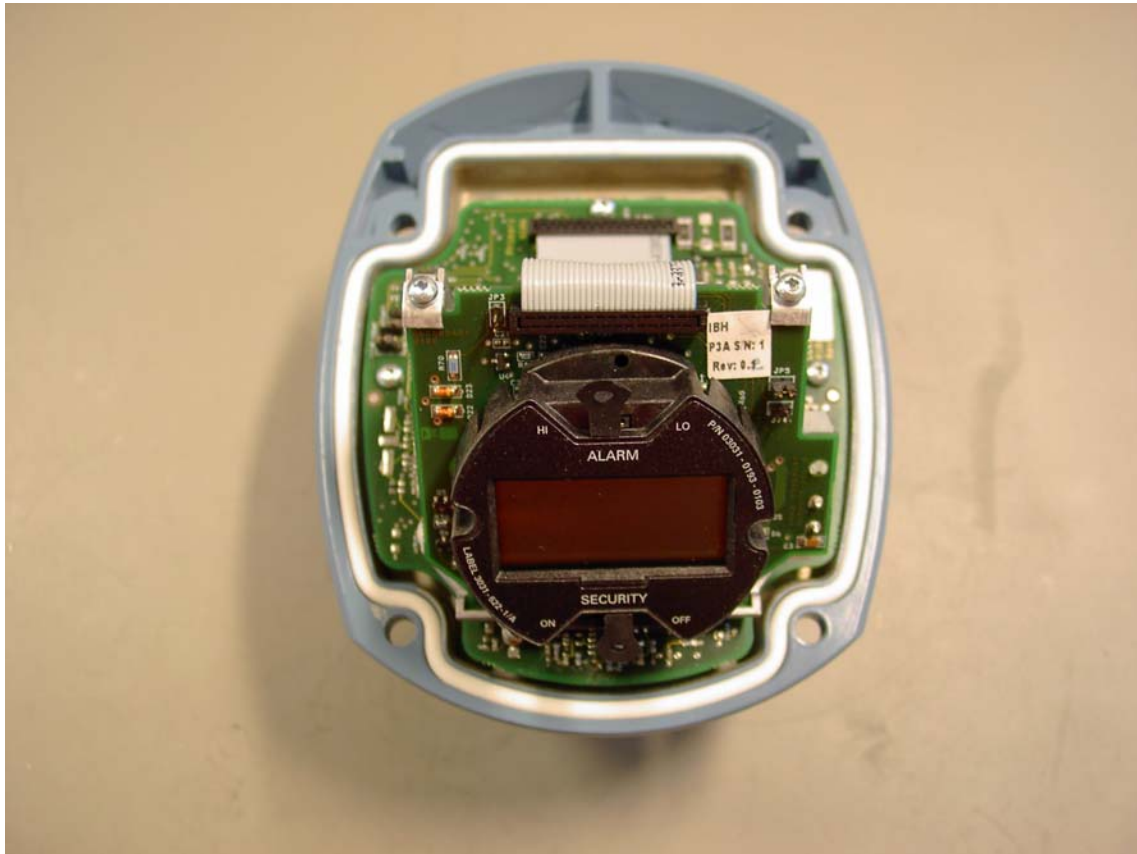
1. Display
