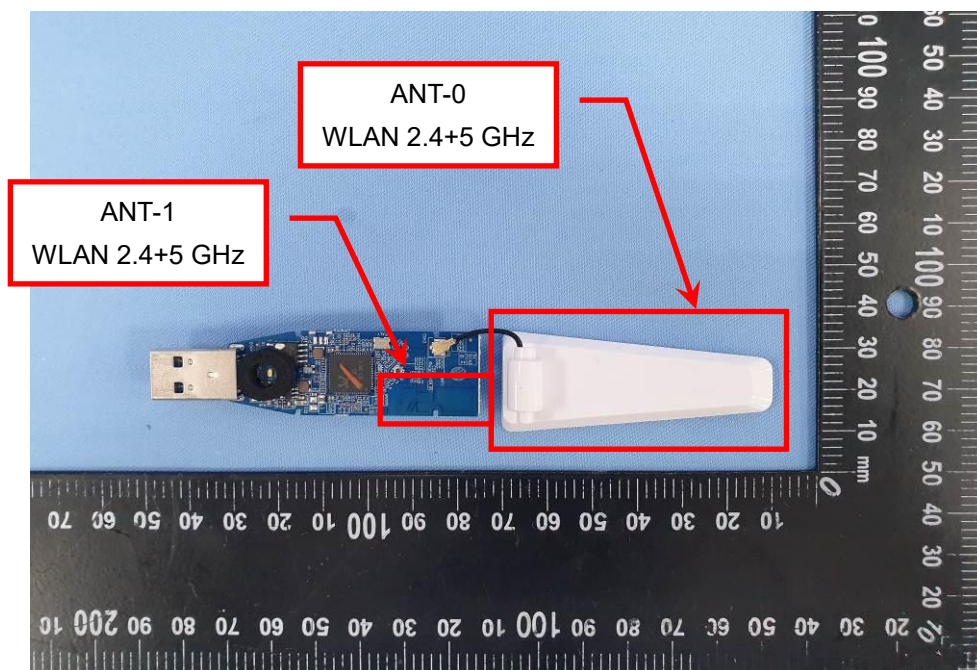
EUT Photo (4)
