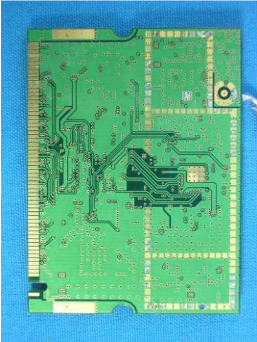
(9) EUT Photo
