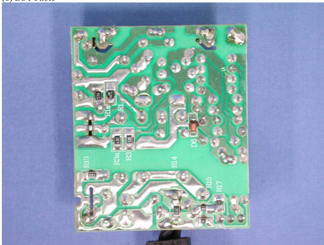
(8) EUT Photo
