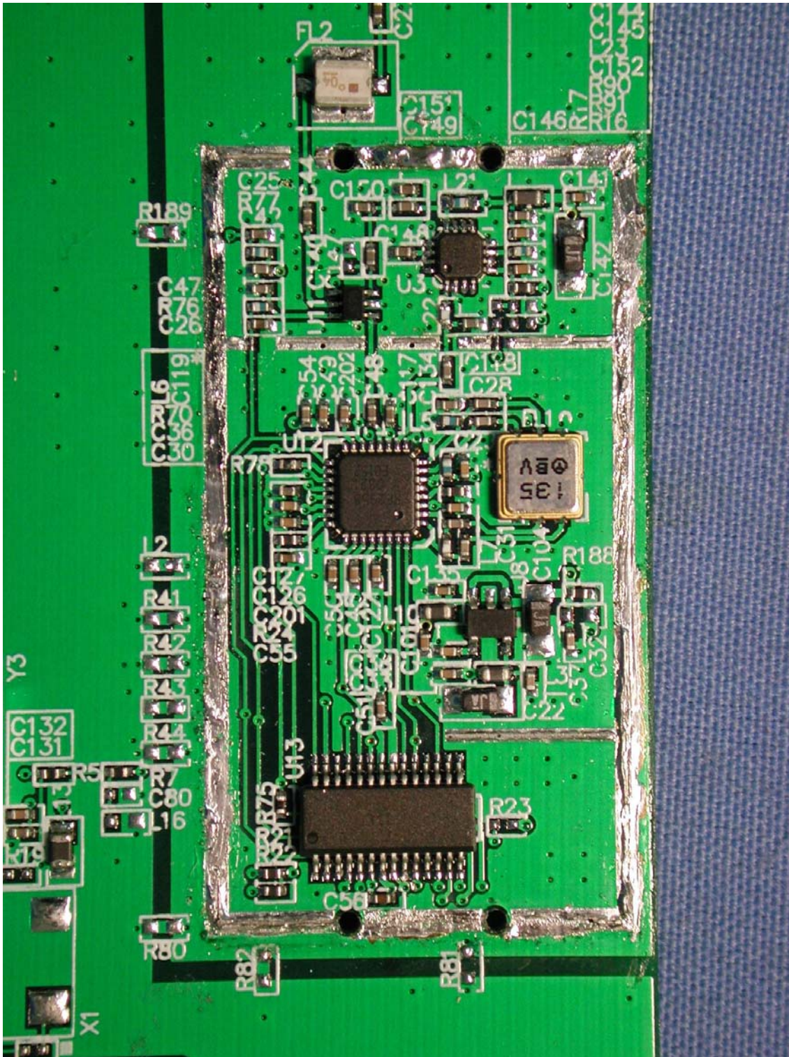
(10) EUT Photo
