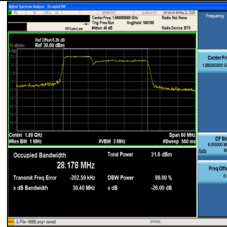
CA_2C-10MHz+20MHz-QPSK-18956+19100- 50RB#0+100RB#0-PASS
