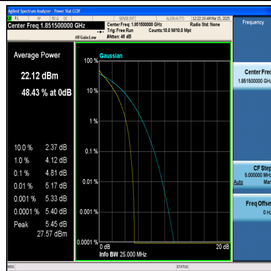
Band2-3MHz-QPSK-18615-15RB#0-PASS
