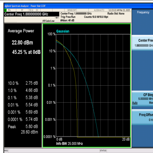
Band2-3MHz-QPSK-18900-15RB#0-PASS
