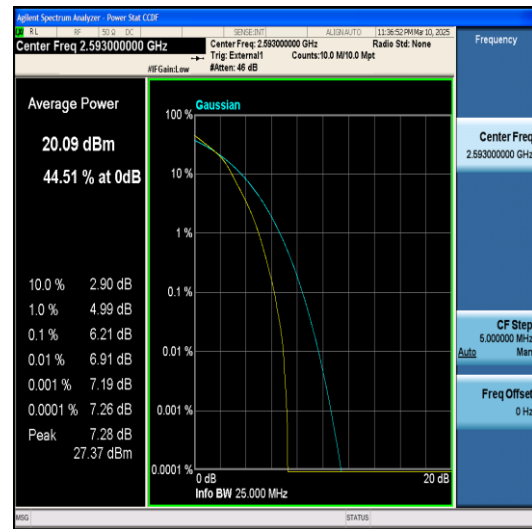
Band41-20MHz-QPSK-41490-1RB#0-PASS
