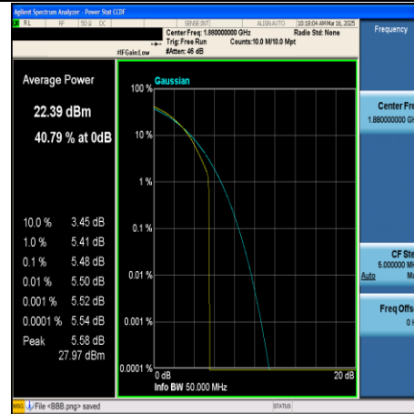
CA_2C-20MHz+20MHz-QPSK-18801+18999- 100RB#0+100RB#0-PASS
