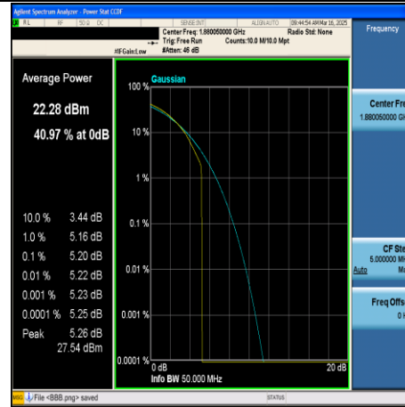
CA_2C-10MHz+20MHz-QPSK-18806+18950- 50RB#0+100RB#0-PASS
