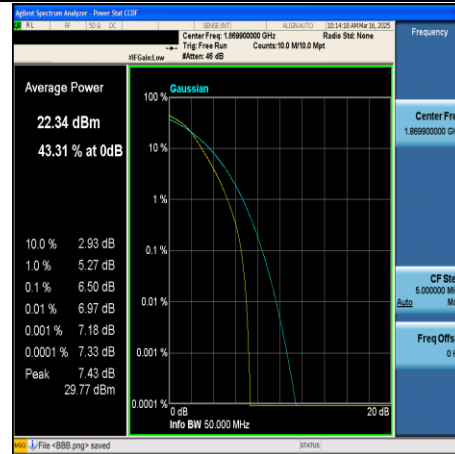
CA_2C-20MHz+20MHz-64QAM-18700+18898- 100RB#0+100RB#0-PASS
