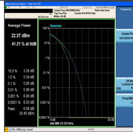
CA_5B-5MHz+10MHz-QPSK-20478+20550- 25RB#0+50RB#0-PASS
