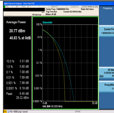
CA_2C-20MHz+20MHz-64QAM-18700+18898- 100RB#0+100RB#0-PASS
