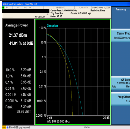
CA_2C-20MHz+20MHz-16QAM-18700+18898- 100RB#0+100RB#0-PASS
