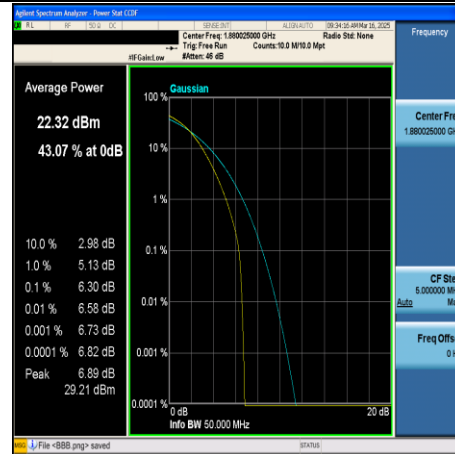
CA_2C-5MHz+20MHz-QPSK-18808+18925- 25RB#0+100RB#0-PASS
