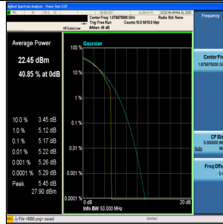
CA_2C-15MHz+20MHz-QPSK-18803+18974- 75RB#0+100RB#0-PASS
