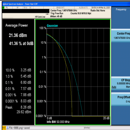
CA_2C-15MHz+20MHz-16QAM-18678+18849- 75RB#0+100RB#0-PASS
