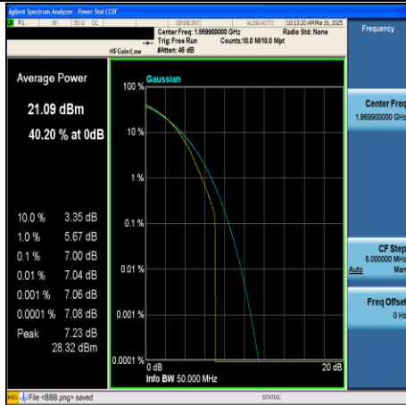
CA_2C-20MHz+20MHz-16QAM-18700+18898- 100RB#0+100RB#0-PASS
