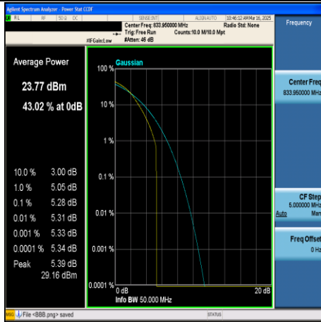
CA_5B-10MHz+10MHz-64QAM-20450+20549- 1RB#49+1RB#0-PASS
