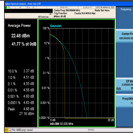
CA_5B-10MHz+10MHz-QPSK-20476+20575- 50RB#0+50RB#0-PASS
