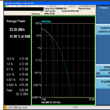
CA_7C-10MHz+20MHz-QPSK-21006+21150- 50RB#0+100RB#0-PASS
