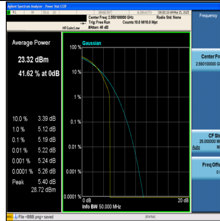
CA_7C-20MHz+20MHz-QPSK-21152+21350- 100RB#0+100RB#0-PASS
