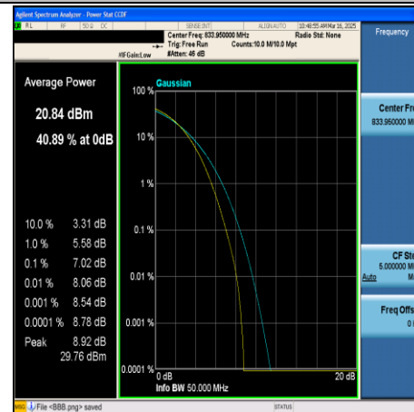
CA_5B-10MHz+10MHz-64QAM-20450+20549- 50RB#0+50RB#0-PASS
