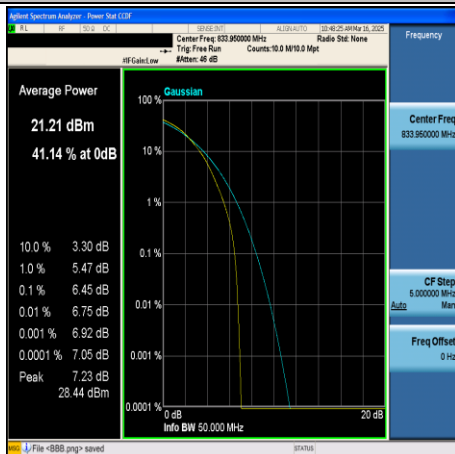
CA_5B-10MHz+10MHz-16QAM-20450+20549- 50RB#0+50RB#0-PASS
