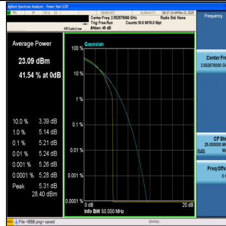
CA_7C-15MHz+20MHz-QPSK-21179+21350- 75RB#0+100RB#0-PASS
