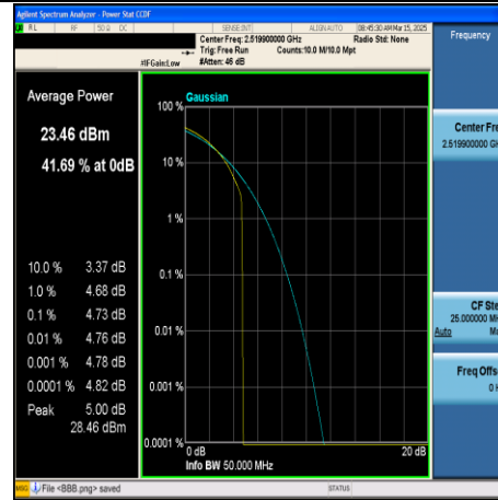
CA_7C-20MHz+20MHz-QPSK-20850+21048- 100RB#0+100RB#0-PASS
