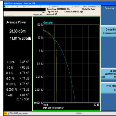
CA_7C-20MHz+20MHz-QPSK-21001+21199- 100RB#0+100RB#0-PASS
