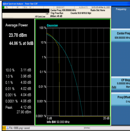
CA_5B-10MHz+10MHz-64QAM-20476+20575- 1RB#49+1RB#0-PASS
