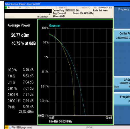
CA_41C-20MHz+20MHz-64QAM-40521+40719- 100RB#0+100RB#0-PASS
