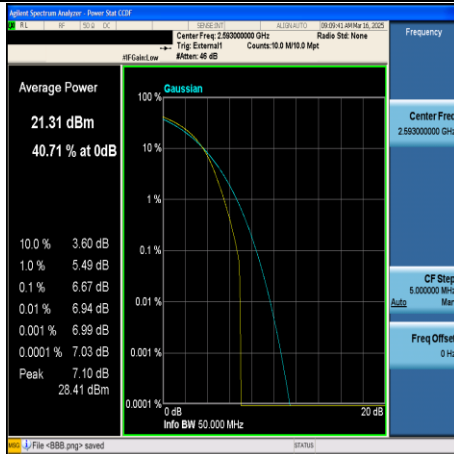
CA_41C-20MHz+20MHz-16QAM-40521+40719- 100RB#0+100RB#0-PASS
