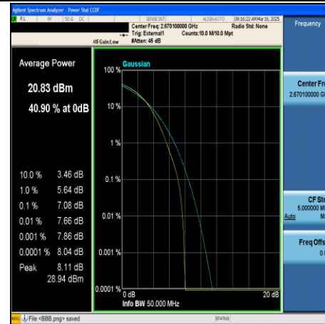
CA_41C-20MHz+20MHz-64QAM-41292+41490- 100RB#0+100RB#0-PASS
