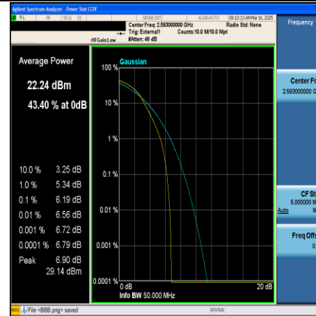
CA_41C-20MHz+20MHz-64QAM-40521+40719- 100RB#0+100RB#0-PASS
