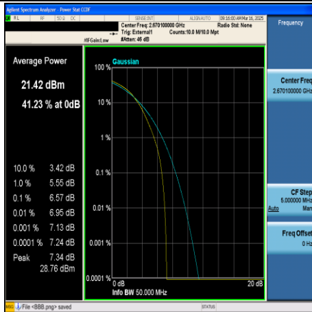
CA_41C-20MHz+20MHz-16QAM-41292+41490- 100RB#0+100RB#0-PASS
