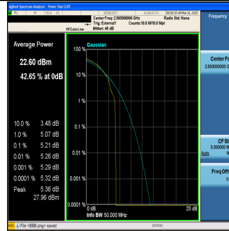
CA_41C-20MHz+20MHz-QPSK-40521+40719- 100RB#0+100RB#0-PASS
