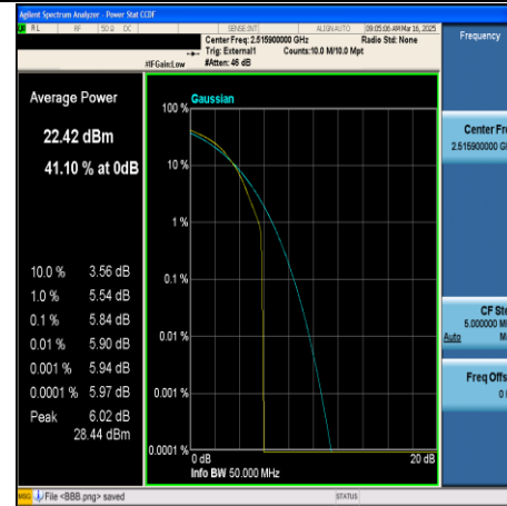
CA_41C-20MHz+20MHz-QPSK-39750+39948- 100RB#0+100RB#0-PASS
