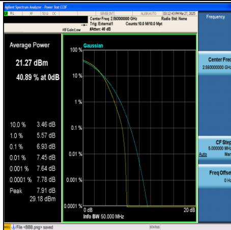
CA_41C-20MHz+20MHz-16QAM-40521+40719- 100RB#0+100RB#0-PASS
