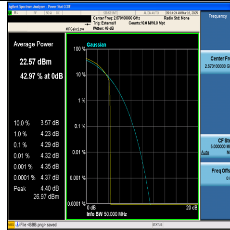
CA_41C-20MHz+20MHz-QPSK-41292+41490- 100RB#0+100RB#0-PASS
