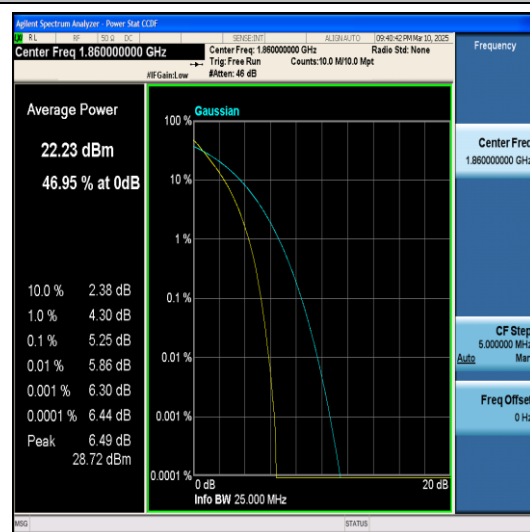
Band2-20MHz-QPSK-18700-100RB#0-PASS
