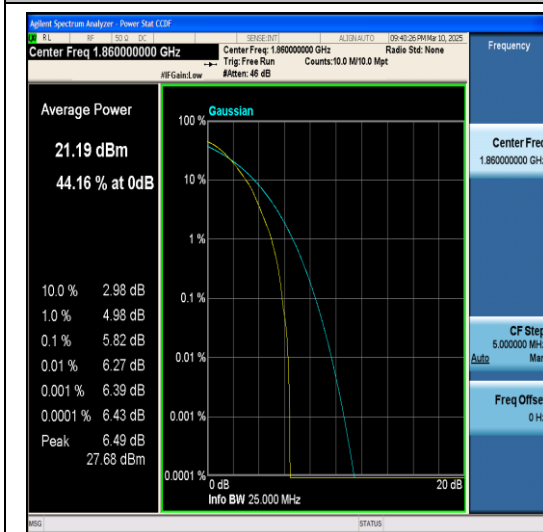
Band2-20MHz-64QAM-18700-1RB#0-PASS
