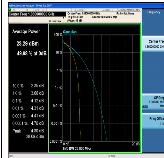
Band2-20MHz-64QAM-18700-1RB#0-PASS
