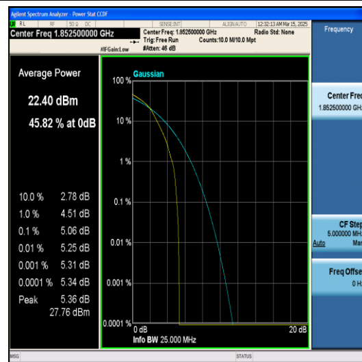
Band2-5MHz-QPSK-18625-25RB#0-PASS
