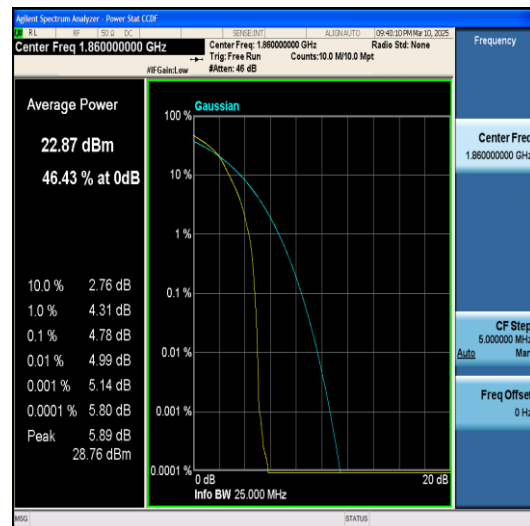
Band2-20MHz-QPSK-18700-100RB#0-PASS
