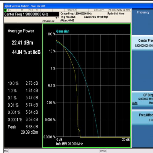
Band2-20MHz-QPSK-19100-100RB#0-PASS
