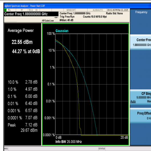
Band2-20MHz-QPSK-18900-100RB#0-PASS
