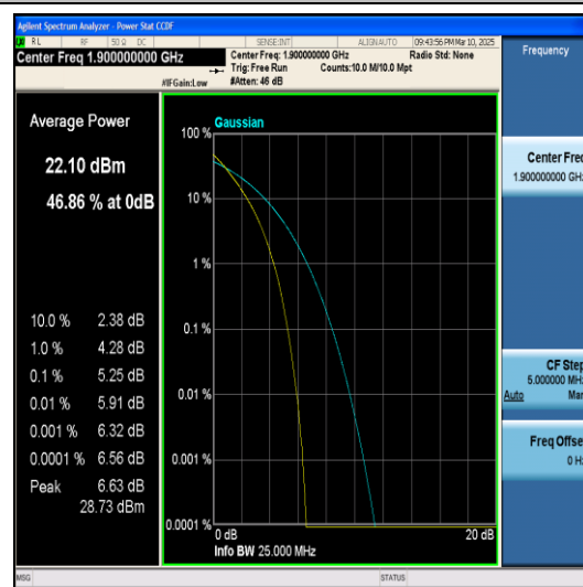
Band2-20MHz-QPSK-19100-100RB#0-PASS
