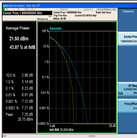
Band2-20MHz-64QAM-18900-1RB#0-PASS
