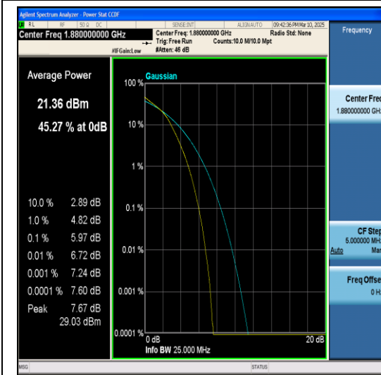
Band2-20MHz-QPSK-19100-1RB#0-PASS
