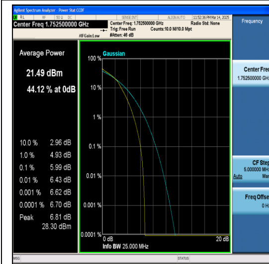
Band4-10MHz-QPSK-20000-1RB#0-PASS
