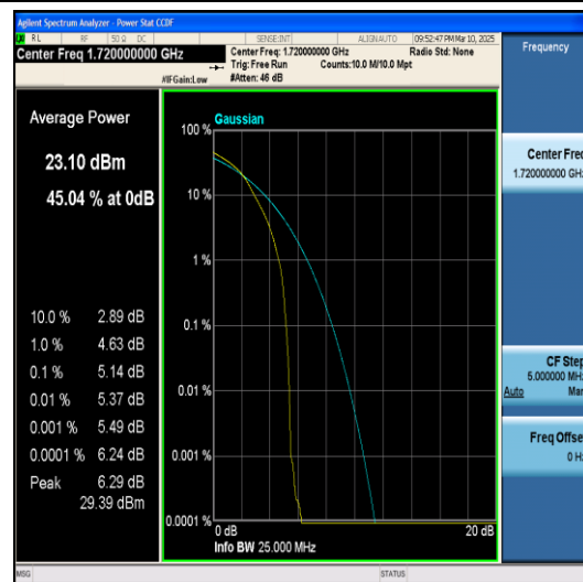
Band4-20MHz-QPSK-20050-100RB#0-PASS
