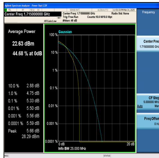
Band4-10MHz-QPSK-20000-50RB#0-PASS
