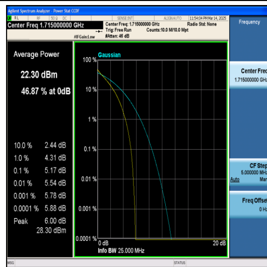
Band4-10MHz-QPSK-20000-50RB#0-PASS
