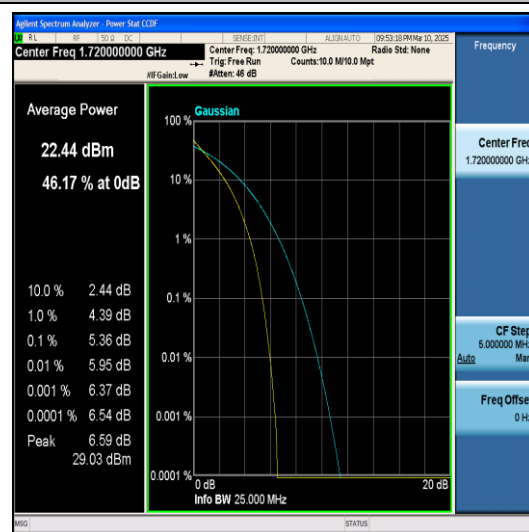
Band4-20MHz-QPSK-20050-100RB#0-PASS
