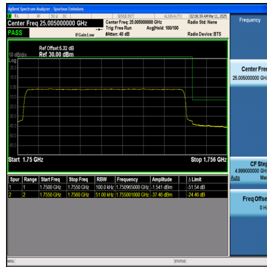
Band4-10MHz-QPSK-20000-1RB#49-PASS
