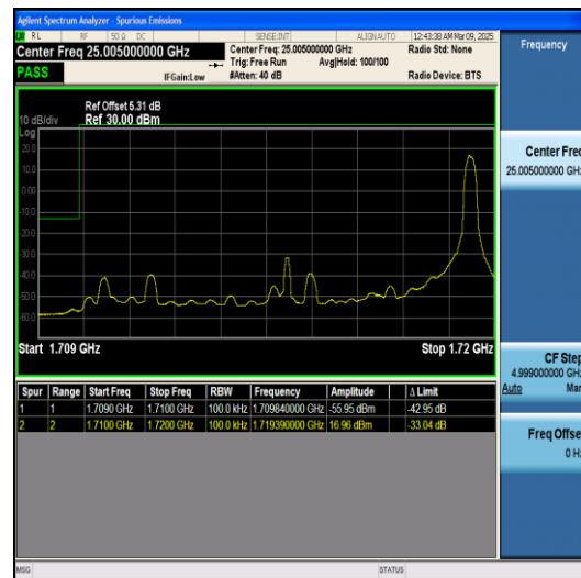
Band4-10MHz-QPSK-20350-1RB#0-PASS
