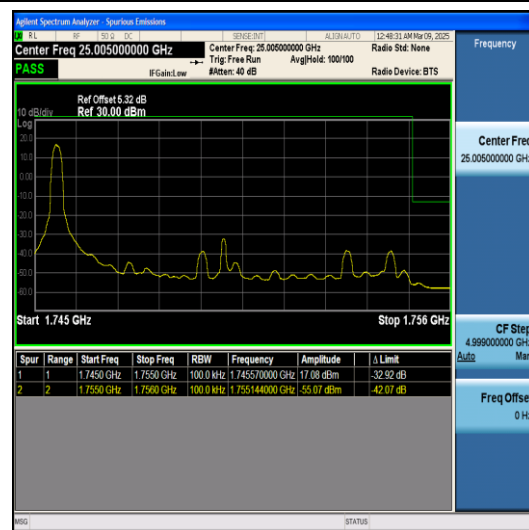
Band4-10MHz-QPSK-20350-1RB#0-PASS
