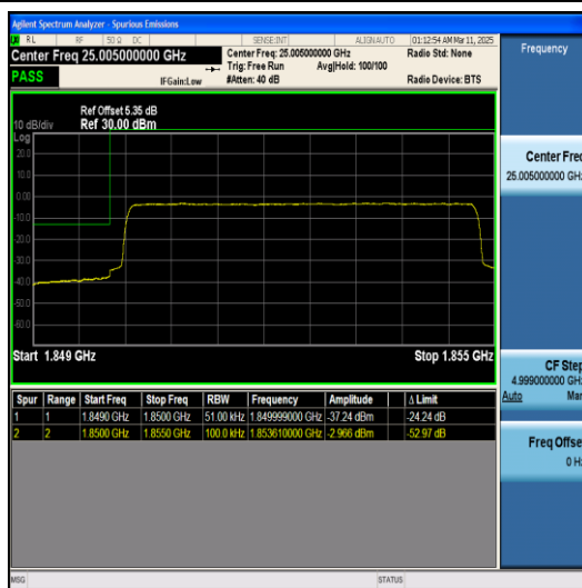
Band2-5MHz-QPSK-18625-25RB#0-PASS
