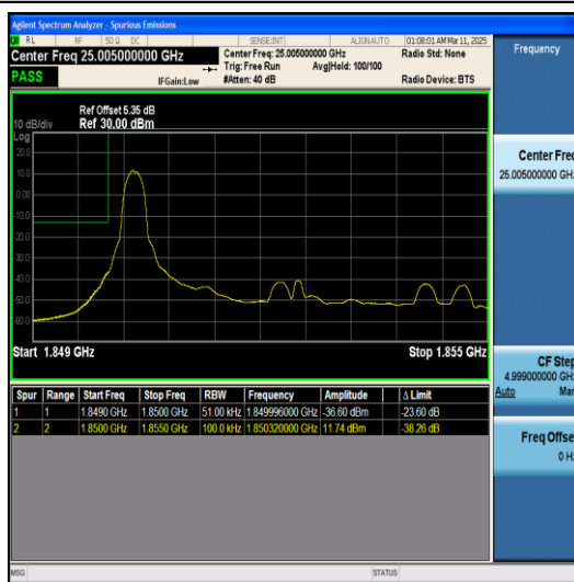
Band2-5MHz-QPSK-18625-25RB#0-PASS
