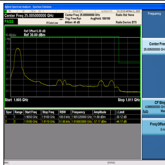
Band2-5MHz-QPSK-19175-1RB#0-PASS
