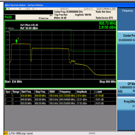
CA_5B-5MHz+10MHz-QPSK-20528+20600- 25RB#0+50RB#0-PASS
