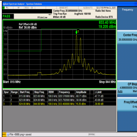
CA_5B-10MHz+10MHz-QPSK-20450+20549- 50RB#0+50RB#0-PASS
