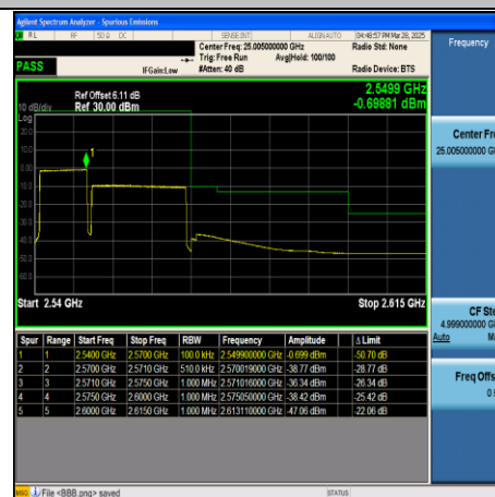
CA_7C-10MHz+20MHz-QPSK-21206+21350- 50RB#0+100RB#0-PASS
