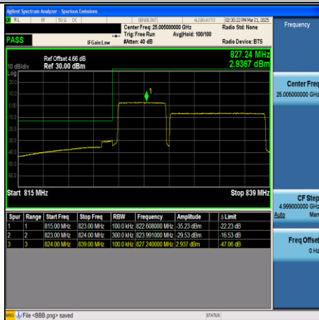
CA_5B-5MHz+10MHz-QPSK-20528+20600- 1RB#0+1RB#49-PASS
