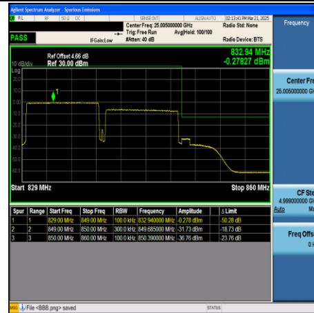
CA_5B-10MHz+10MHz-QPSK-20501+20600- 50RB#0+50RB#0-PASS
