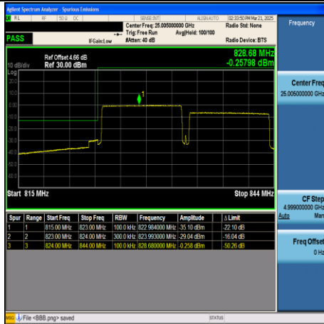
CA_5B-10MHz+10MHz-QPSK-20501+20600- 1RB#0+1RB#49-PASS
