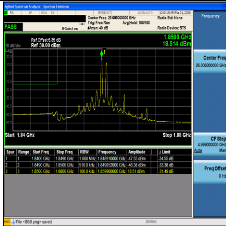
CA_2C-10MHz+20MHz-QPSK-18655+18799- 50RB#0+100RB#0-PASS
