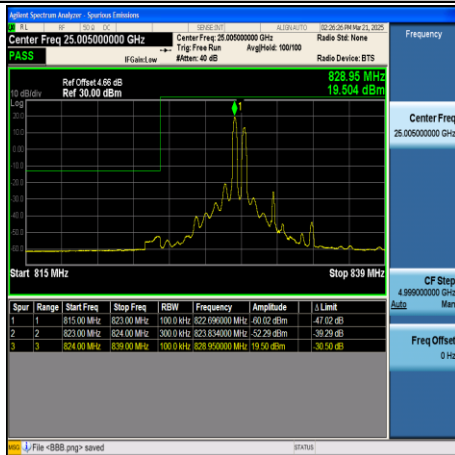
CA_5B-5MHz+10MHz-QPSK-20428+20500- 25RB#0+50RB#0-PASS
