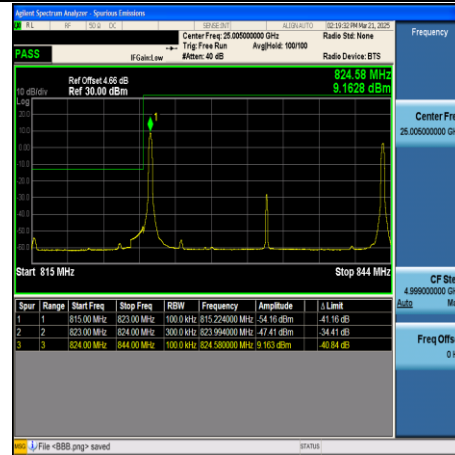
CA_5B-10MHz+10MHz-QPSK-20501+20600- 1RB#49+1RB#0-PASS
