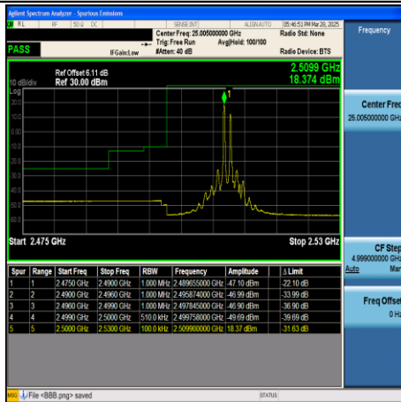
CA_7C-10MHz+20MHz-QPSK-20805+20949- 50RB#0+100RB#0-PASS
