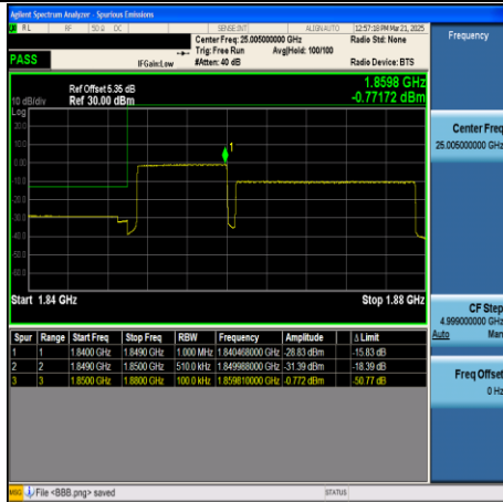
CA_2C-10MHz+20MHz-QPSK-18956+19100- 1RB#0+1RB#99-PASS
