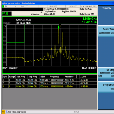
CA_2C-20MHz+20MHz-QPSK-18700+18898- 100RB#0+100RB#0-PASS
