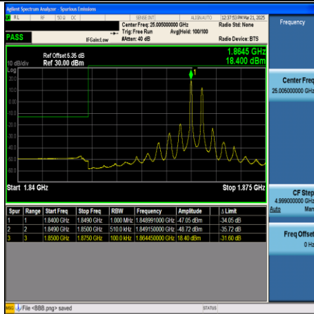
CA_2C-15MHz+20MHz-QPSK-18678+18849- 75RB#0+100RB#0-PASS
