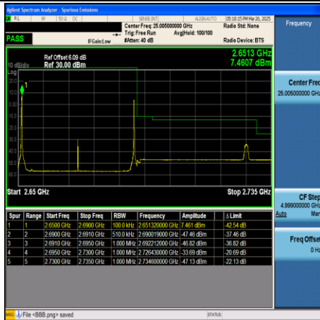
CA_41C-20MHz+20MHz-QPSK-41292+41490- 1RB#0+1RB#99-PASS
