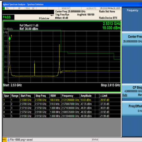
CA_7C-20MHz+20MHz-QPSK-21152+21350- 1RB#0+1RB#99-PASS
