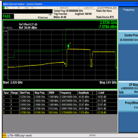
CA_38C-20MHz+20MHz-QPSK-37952+38150- 1RB#0+1RB#99-PASS
