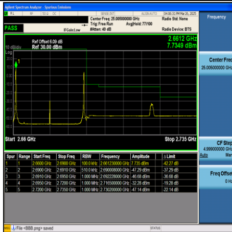
CA_41C-10MHz+20MHz-QPSK-41346+41490- 1RB#0+1RB#99-PASS
