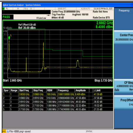
CA_41C-5MHz+20MHz-QPSK-41373+41490- 1RB#0+1RB#99-PASS
