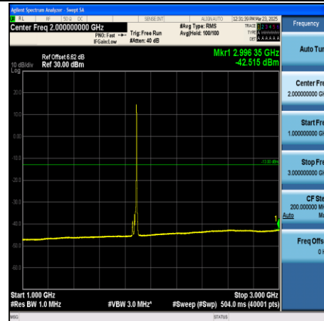
CA_2C-20MHz+20MHz-QPSK-18801+18999- 1RB#99+1RB#0-1000~3000-PASS
