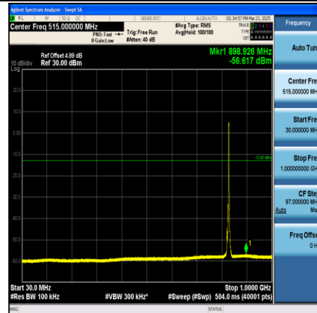
CA_5B-10MHz+10MHz-QPSK-20450+20549- 1RB#49+1RB#0-30~1000-PASS
