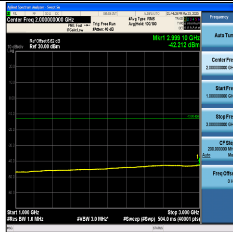
CA_5B-10MHz+10MHz-QPSK-20476+20575- 1RB#49+1RB#0-1000~3000-PASS
