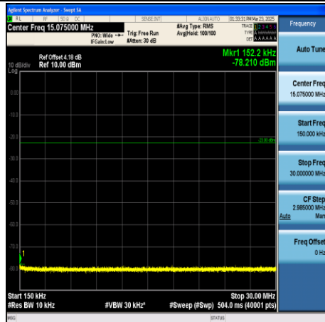
CA_5B-10MHz+10MHz-QPSK-20450+20549- 1RB#49+1RB#0-0.15~30-PASS
