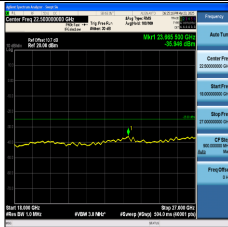
CA_41C-20MHz+20MHz-QPSK-41292+41490- 1RB#99+1RB#0-18000~27000-PASS
