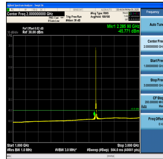
Band40(2305-2320)-10MHz-QPSK-38775-1RB#0- 1000~3000-PASS
