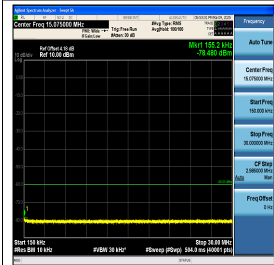
Band40(2305-2320)-10MHz-QPSK-38800-1RB#0- 0.15~30-PASS
