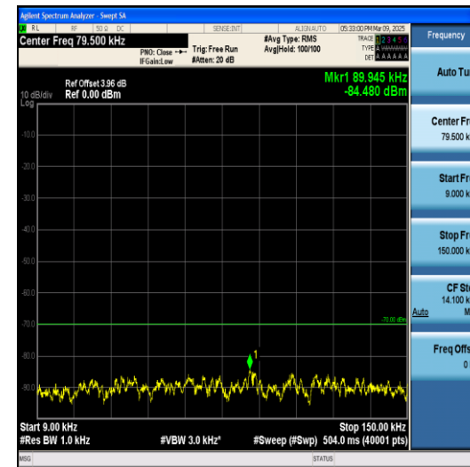
Band40(2305-2320)-5MHz-QPSK-38825-1RB#0-0. 009~0.15-PASS
