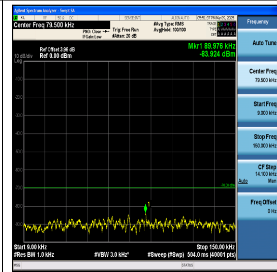
Band40(2305-2320)-10MHz-QPSK-38800-1RB#0- -0.009~0.15-PASS
