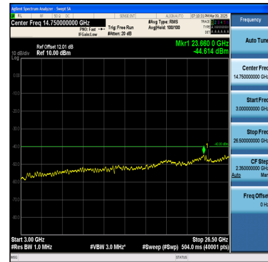
Band40(2305-2320)-10MHz-QPSK-38750-1RB#0- 3000~26500-PASS
