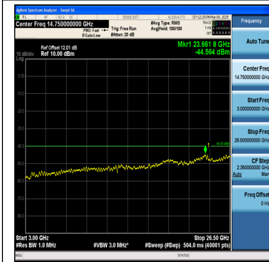
Band40(2305-2320)-10MHz-QPSK-38775-1RB#0- 3000~26500-PASS
