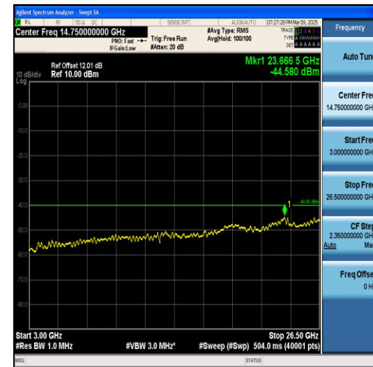
Band40(2345-2360)-10MHz-QPSK-39150-1RB#0- 3000~26500-PASS
