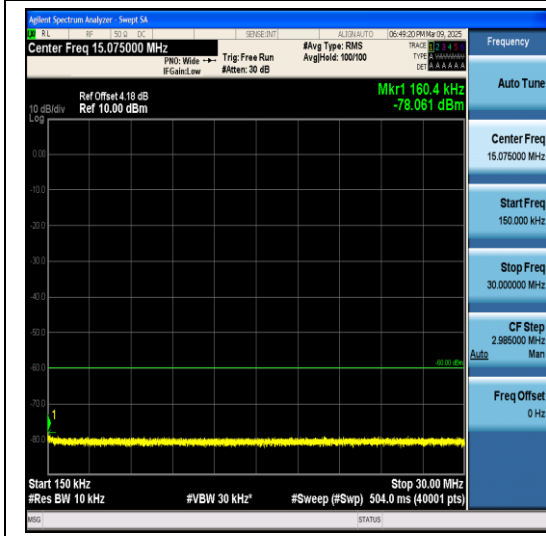
Band40(2345-2360)-10MHz-QPSK-39200-1RB#0- 0.15~30-PASS
