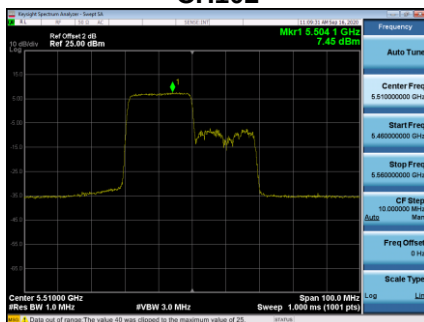
CH102
