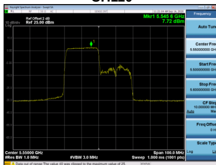
CH110
