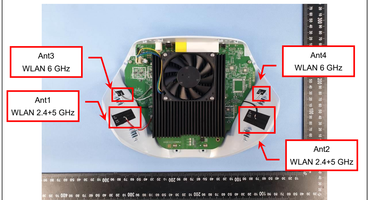
EUT Photo (2)
