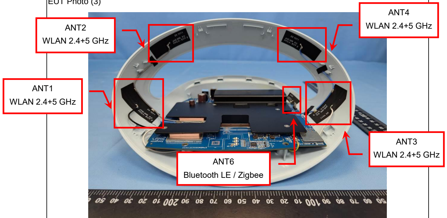
EUT Photo (4)
