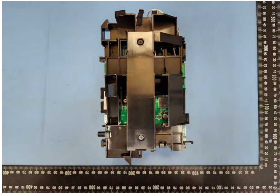
EUT Photo (31)
