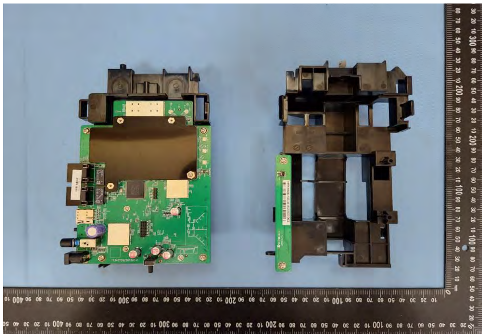
EUT Photo (49)
