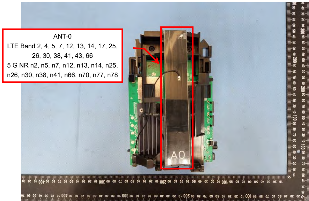
EUT Photo (37)
