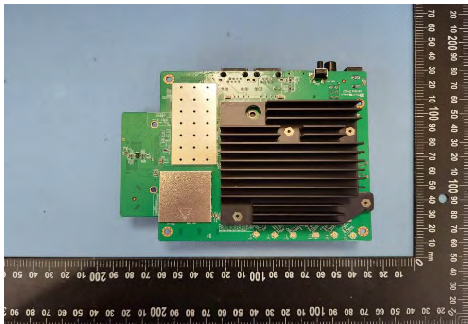
EUT Photo (59)
