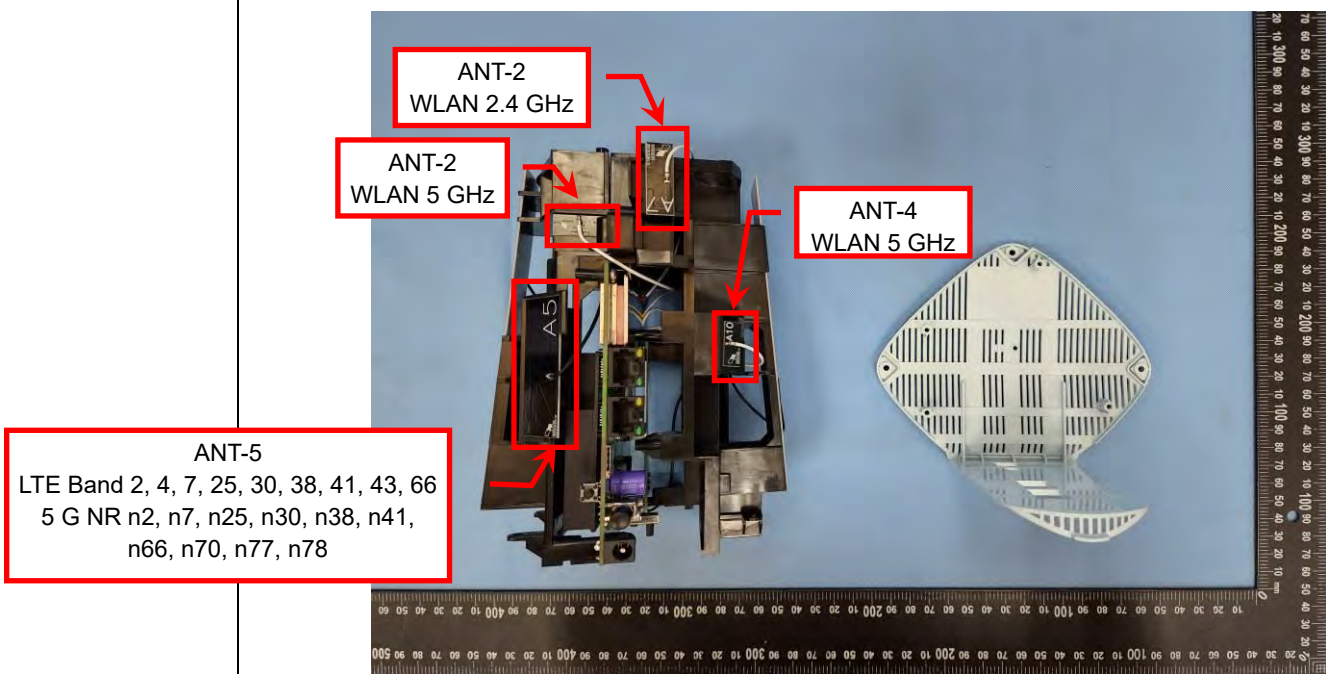
EUT Photo (3)
