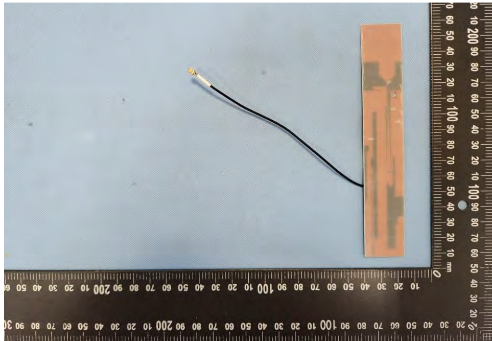
EUT Photo (41)
