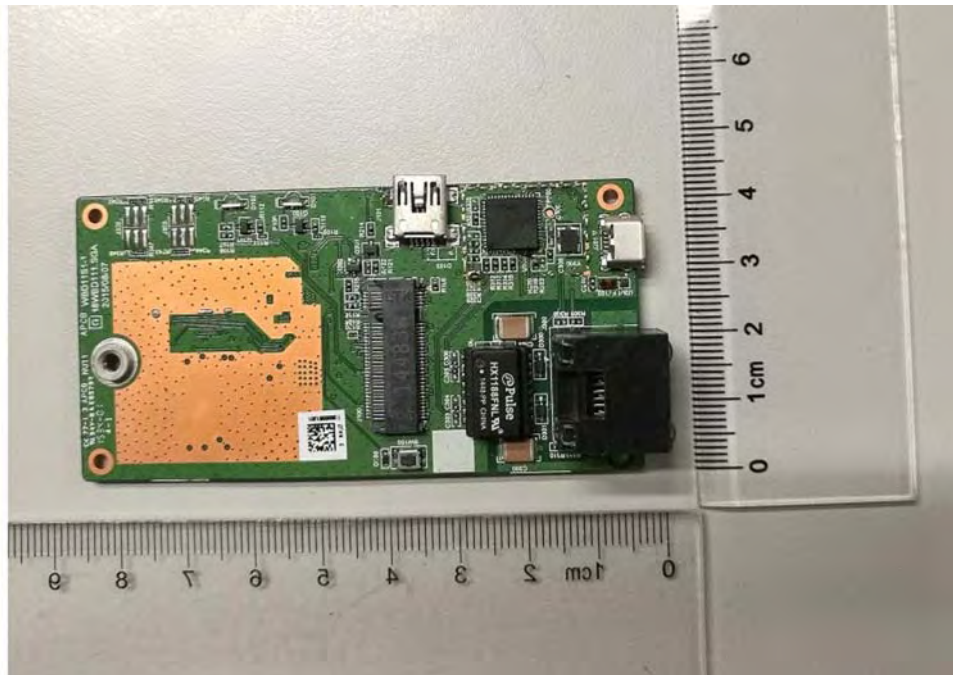
EUT Photo 8 )
