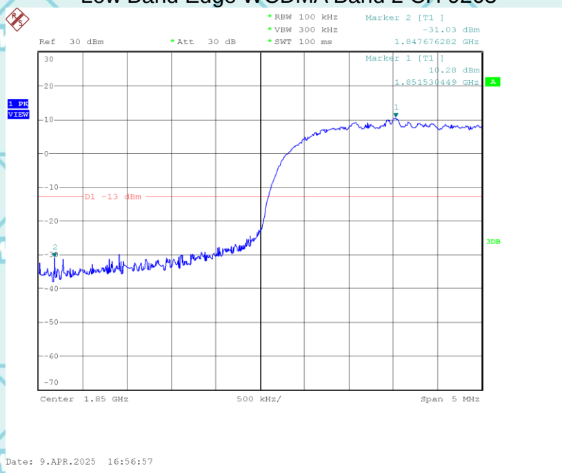
Low Band Edge WCDMA Band 2 CH 9263
