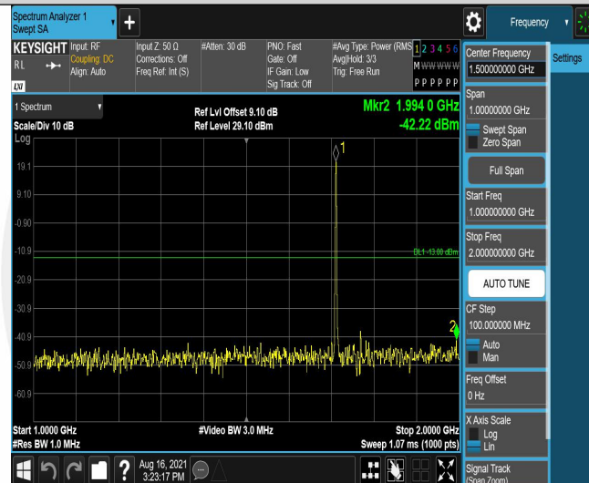
Band4-1.4MHz-16QAM-19957-6RB#0-Range2:1000~2000MHz
