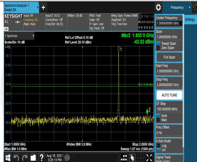
Band4-1.4MHz-QPSK-20393-6RB#0-Range2:1000~2000MHz
