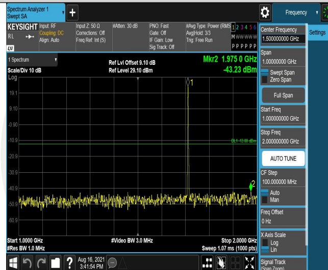
Band4-3MHz-16QAM-19965-6RB#0-Range2:1000~2000MHz
