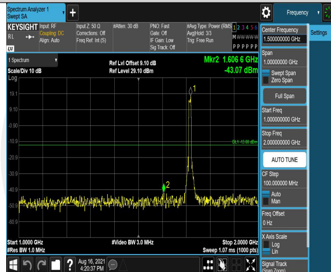
Band4-10MHz-16QAM-20000-50RB#0-Range2:1000~2000MHz
