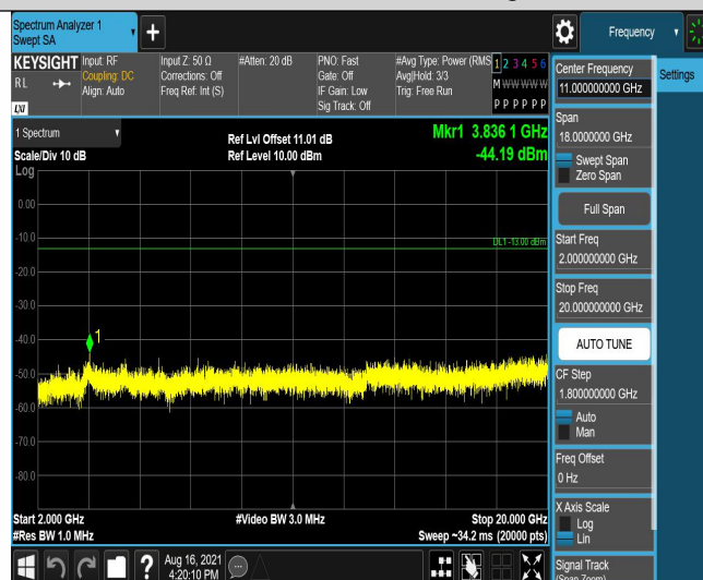
Band4-10MHz-QPSK-20000-50RB#0-Range3:2000~20000MHz
