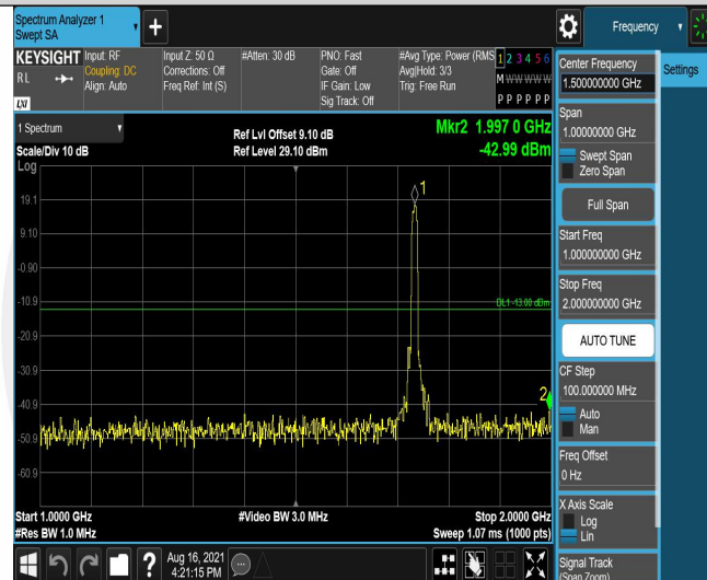
Band4-10MHz-QPSK-20175-50RB#0-Range2:1000~2000MHz
