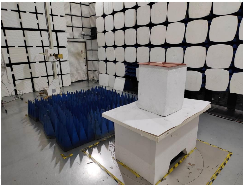
Fig. 2 (Above 1GHz)
