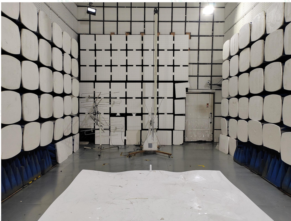
Fig. 1 (30MHz~1GHz)
