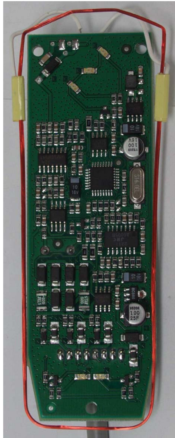
PCB-Top
