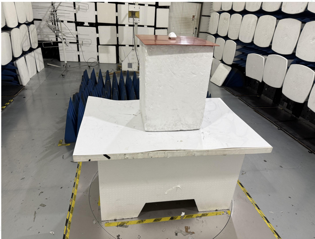
Fig. 3 (Above 1GHz)
