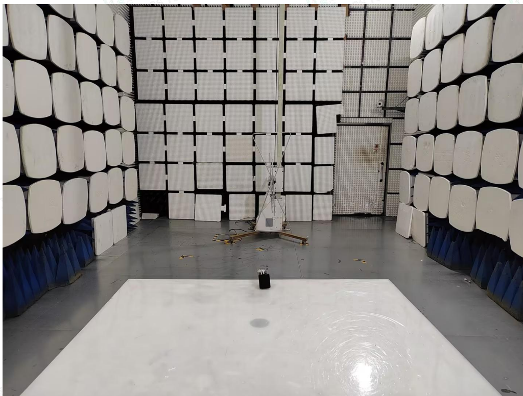
Fig. 1 (30MHz~1GHz)
