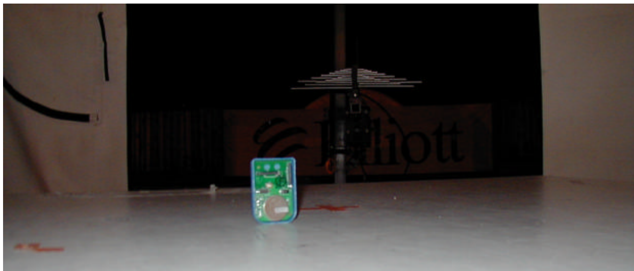
EUT Upright
